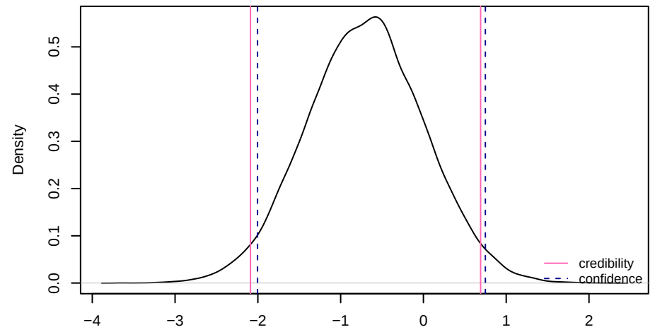
Posterior Density of \beta_1
