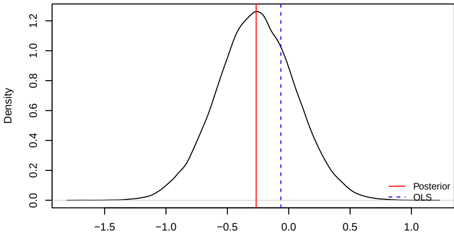
Posterior Density of \beta_4
