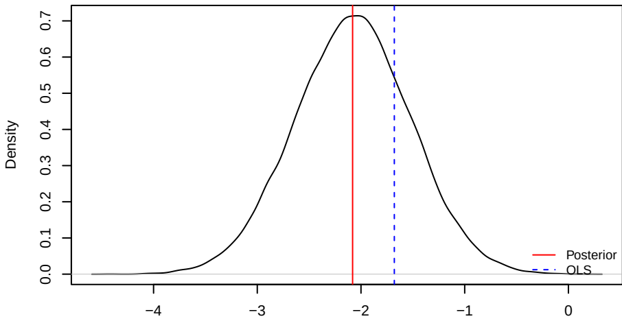
Posterior Density of \beta_2
