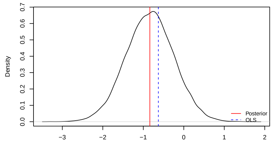
Posterior Density of \beta_1
