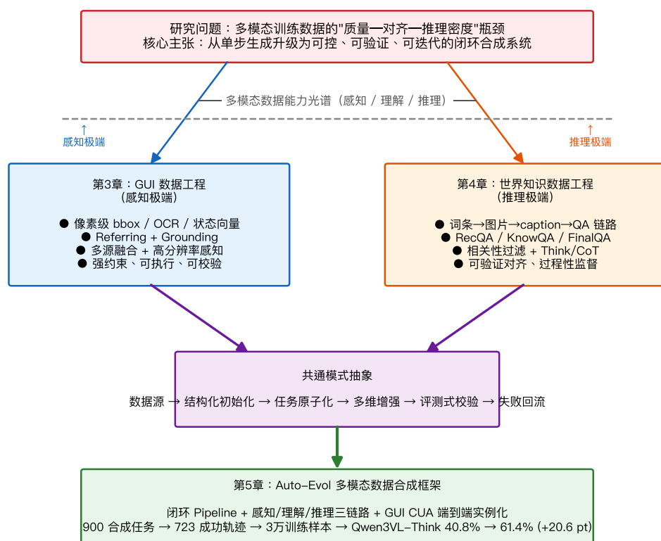
图 1-1 本文研究架构概览：上层为研究问题与核心主张；中部为“数据能力光谱”两极——第3章 GUI 数据工程（感知极端）与第4章世界知识数据工程（推理极端）；下层为从两极归纳的共通骨架及其抽象为 Auto-Evol 框架（第5章），并以 GUI CUA 端到端 SFT 实验验证。
