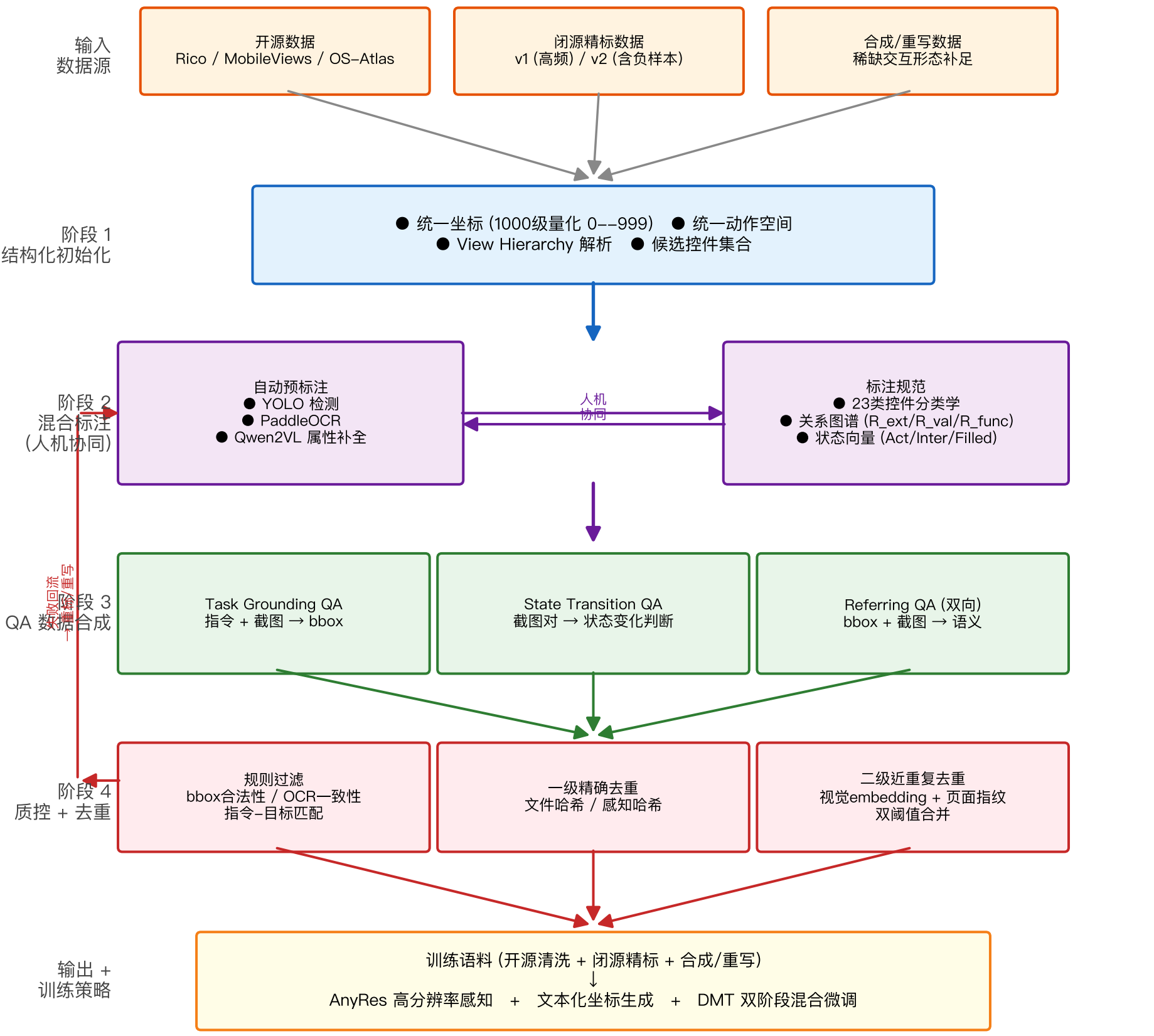
图：GUI 数据合成流水线 (4阶段 + 失败回流闭环)
