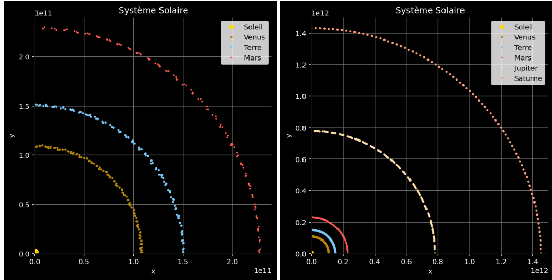
FIGURE 7 – Zoom sur la trajectoire des planètes Tellurique et de Jupiter et Saturne
