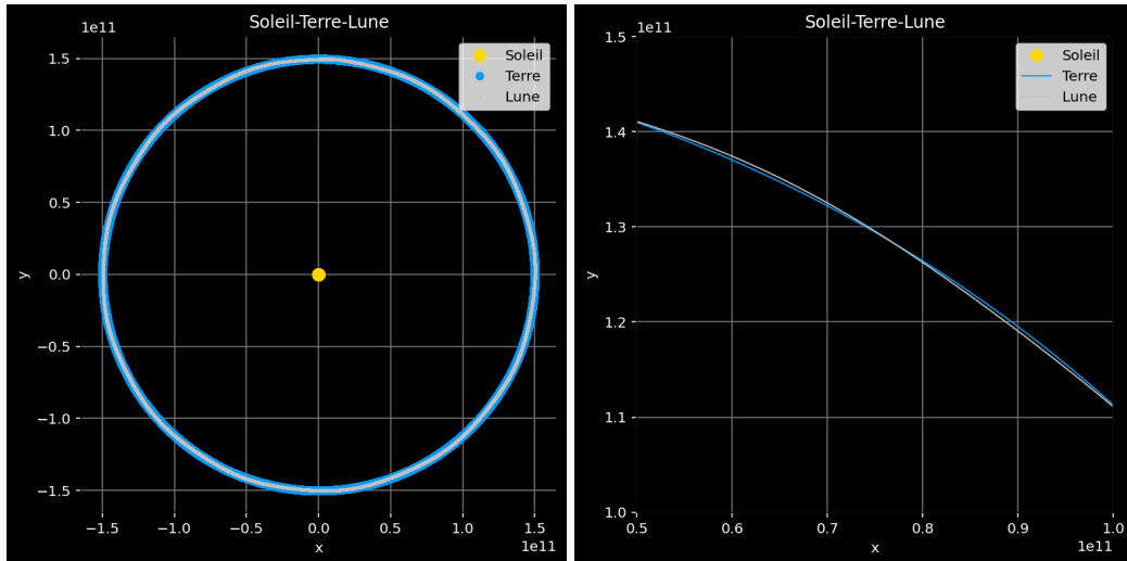
FIGURE 1 – Trajectoires de la Lune et de la Terre autour du Soleil & Zoom
