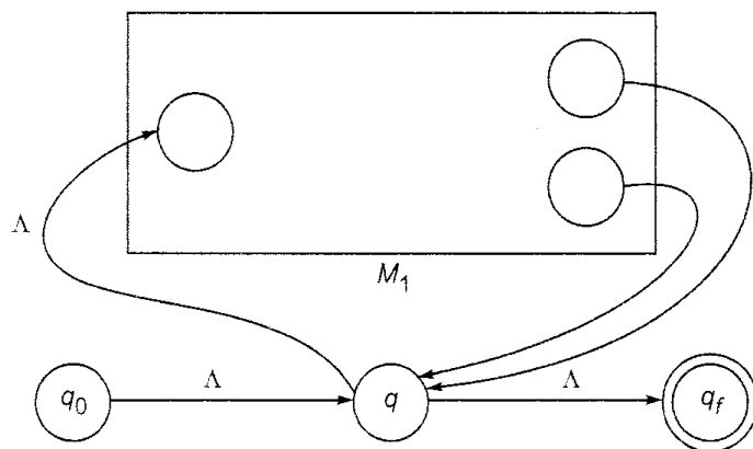
Fig. 5.9 NFA accepting L(P^*) .
