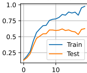
Mem size : 526
