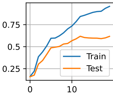
Mem size : 526
