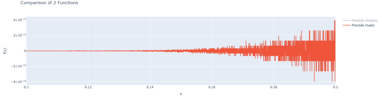
Figura 2.7: Comportamento da expressão f(x) = (x \times x \times x \times x \times x \times x \times x \times x \times x \times x) - x^{10} , com precisão dupla, no intervalo [0,1,0,2] .
