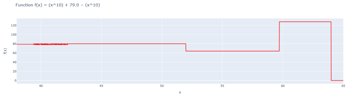
Figura 2.4: Comportamento da expressão x^{10} + 79 - x^{10} no intervalo [38, 65] .
