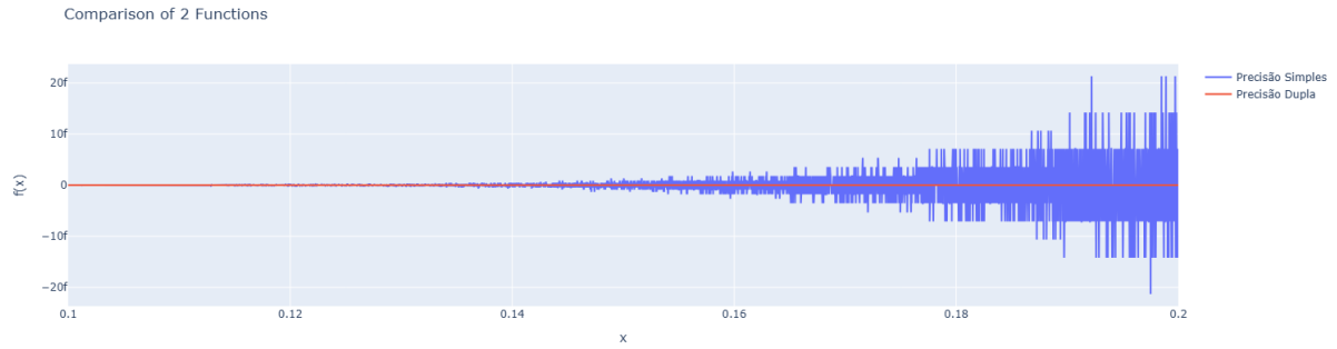
Figura 2.8: Comportamento da expressão f(x) = (x \times x \times x \times x \times x \times x \times x \times x \times x \times x) - x^{10} , com precisão simples, no intervalo [0,1,0,2] .
