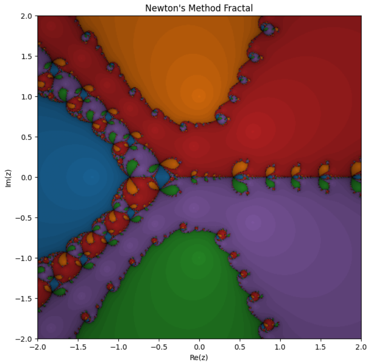
Figura 3.17: Fractais de Newton - Polinomio ABCD.
