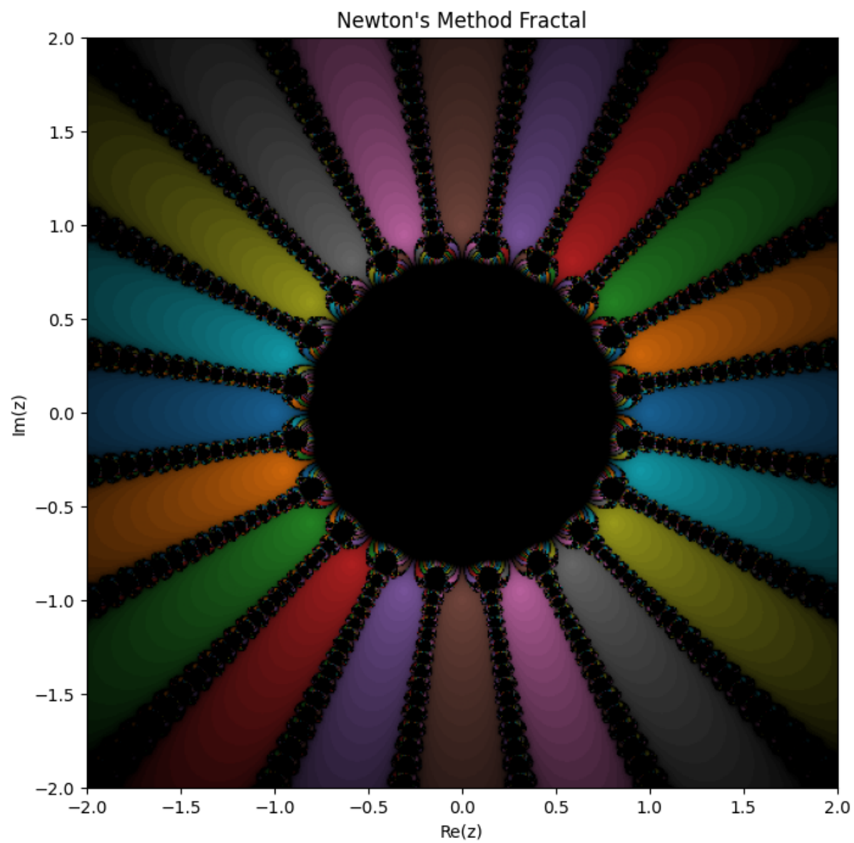
Figura 3.15: Fractais de Newton - 20 Unidades da raiz.
