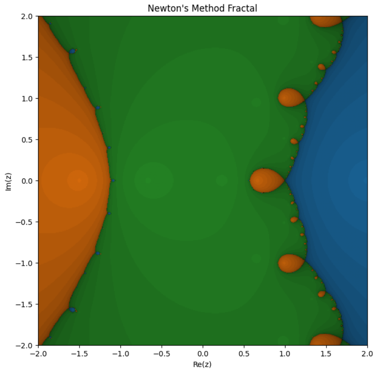
Figura 3.18: Fractais de Newton - Polinomio ABCD.
