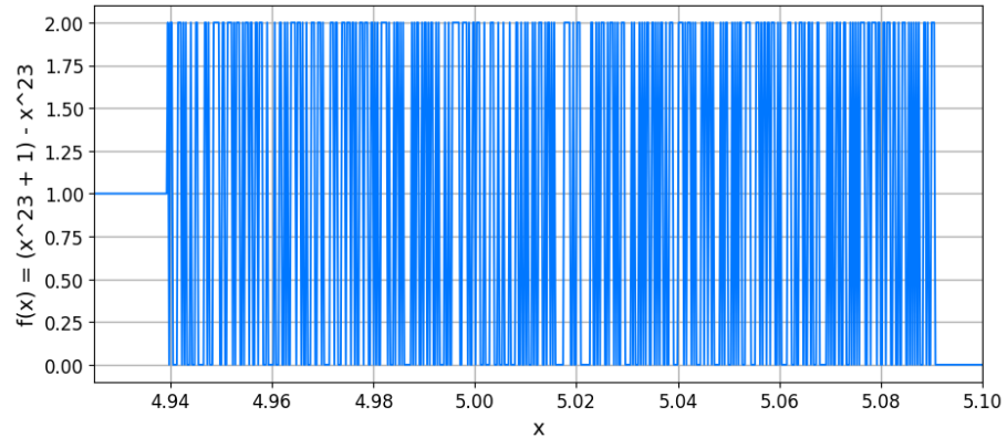
Figura 2: Resultado da avaliação da função f(x) = x^{23} + 1 - x^{23} num SPF IEEE de 64 bits. Fonte: Autor.
