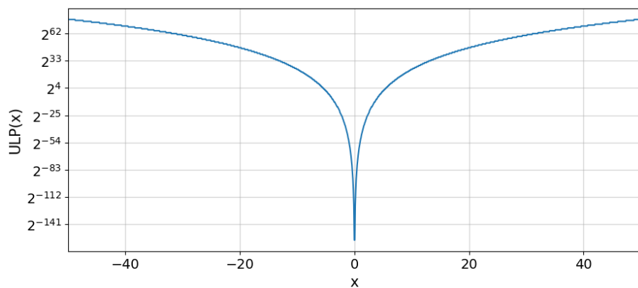
Figura 1: Gráfico da Função ULP(x^{23}) num SPF IEEE de 64 bits. Fonte: Autor.
