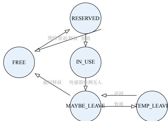
图 7 座位状态机
