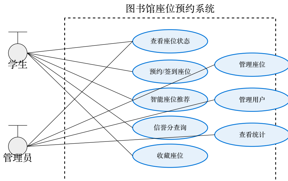
图 1 系统用例图
