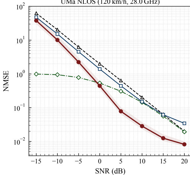
UMa NLOS (120 km/h, 28.0 GHz)
