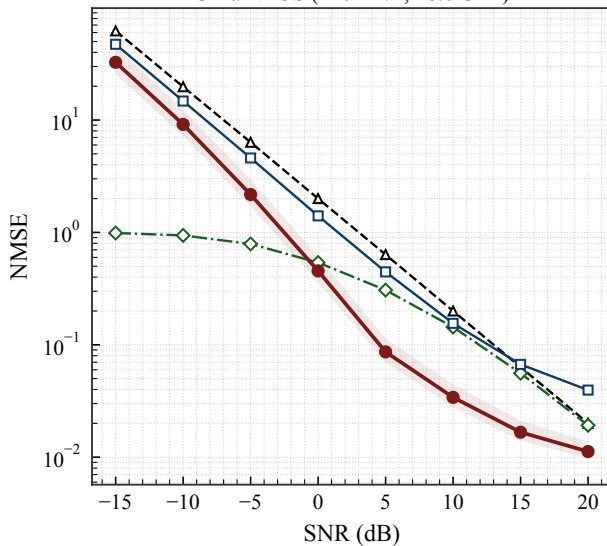
UMa NLOS (120 km/h, 28.0 GHz)
