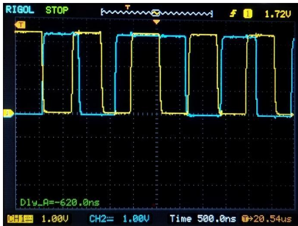
Gambar 4-4-2 Osiloskop Percobaan 4 saat Frekuensi melebihi batas (800 kHz)
