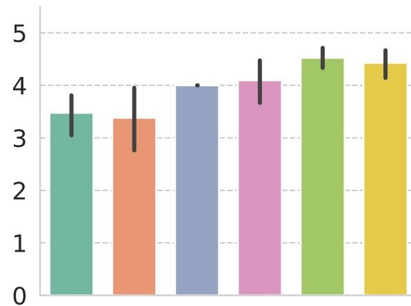
Gemma 3 (1B)
