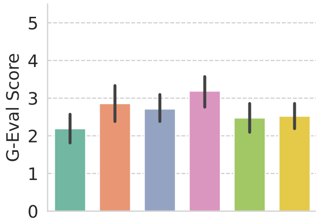
Llama 3.2 (1B)
