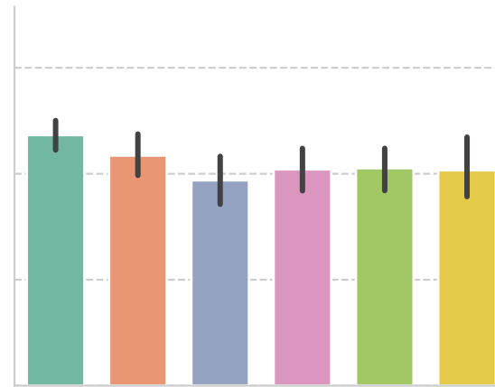
Gemma 3 (1B)
