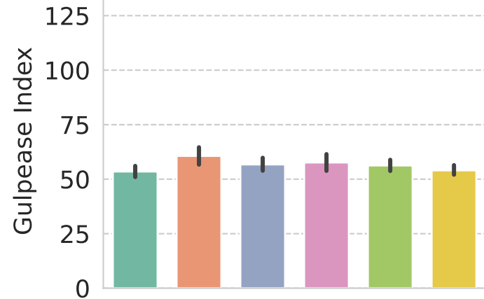
Llama 3.2 (1B)
