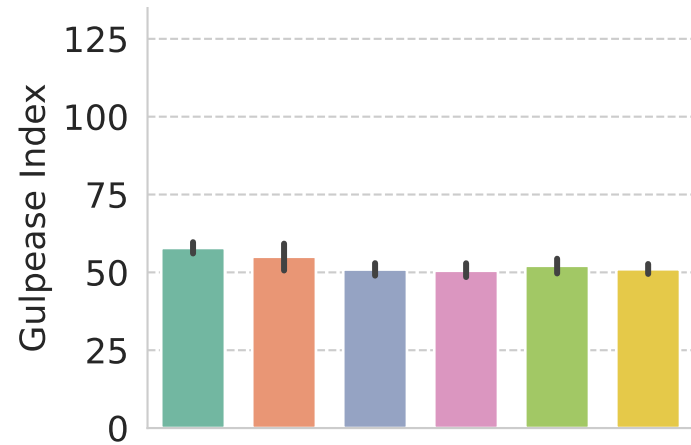
Llama 3.2 (1B)
