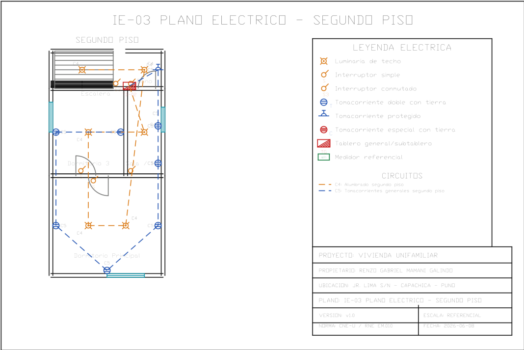
Figura 7.2: Plano de Instalaciones Eléctricas - Segundo Piso
