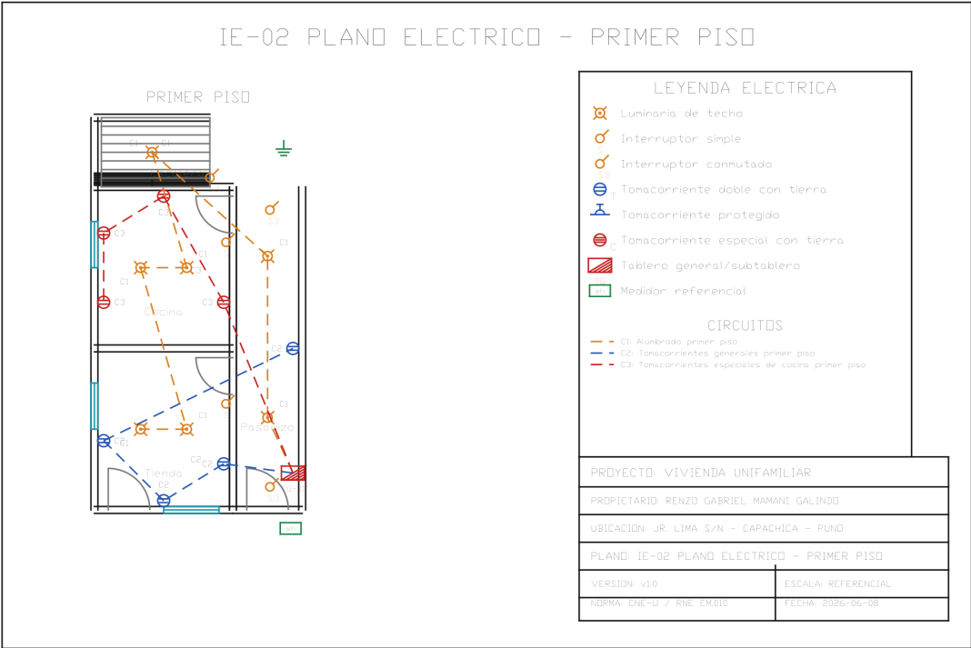
Figura 7.1: Plano de Instalaciones Eléctricas - Primer Piso
