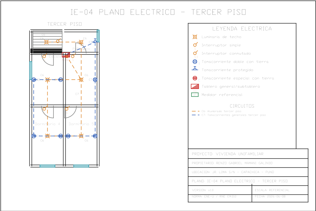
Figura 7.3: Plano de Instalaciones Eléctricas - Tercer Piso
