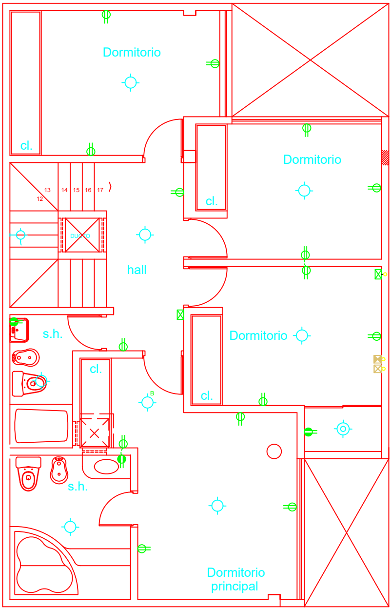
SEGUNDO PISO
