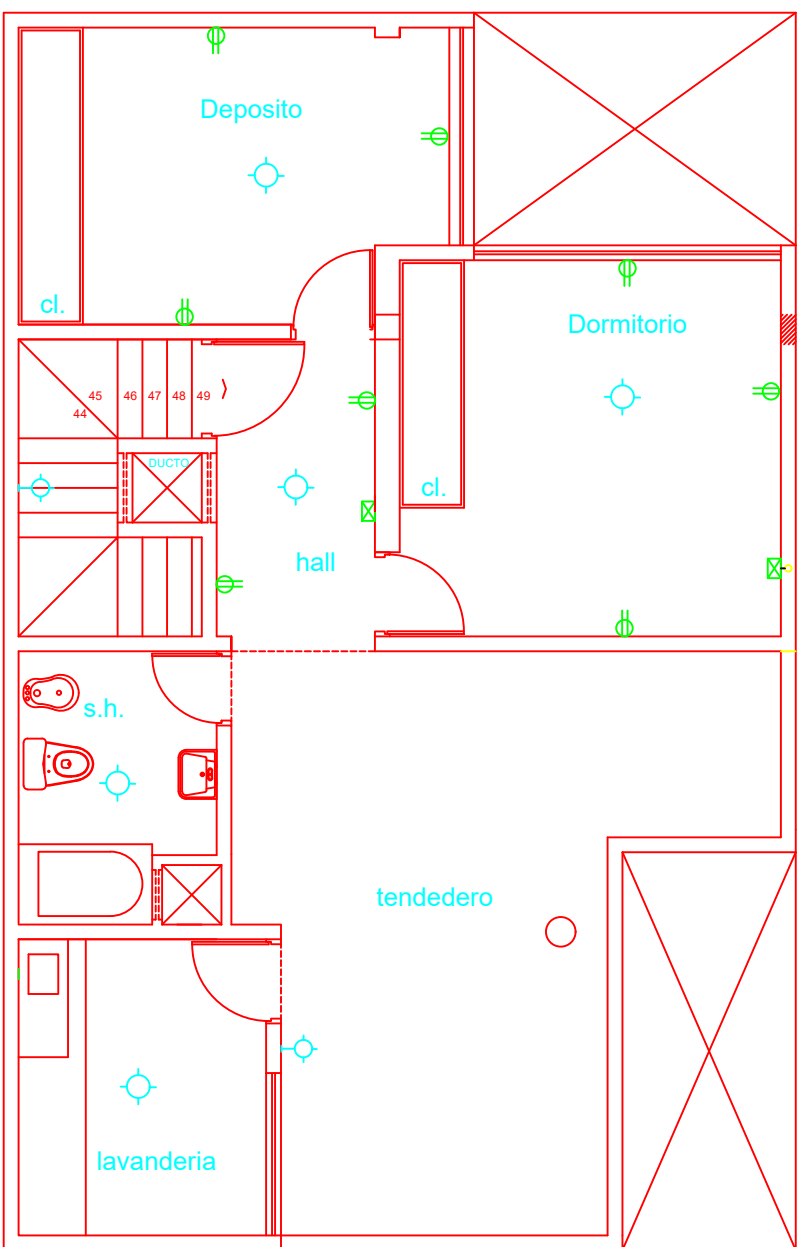
AZOTEA
