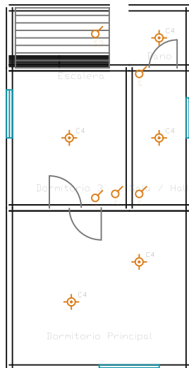
SEGUNDO PISO
