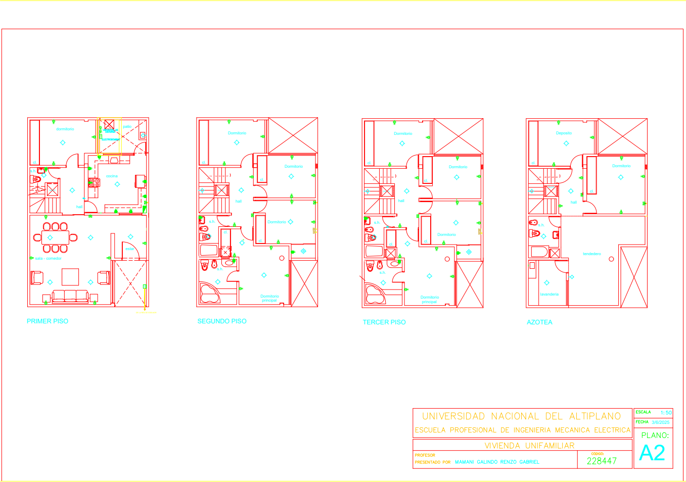
Figura 7.1: Avance del plano eléctrico de la vivienda (Alumbrado y Tomacorrientes)
