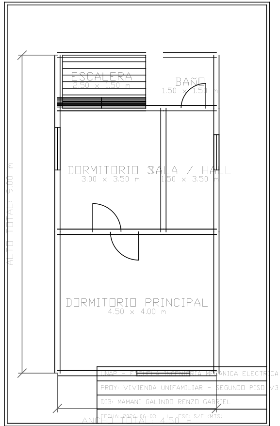
Figura 7.3: Plano de Distribución Arquitectónica - Segundo Piso
