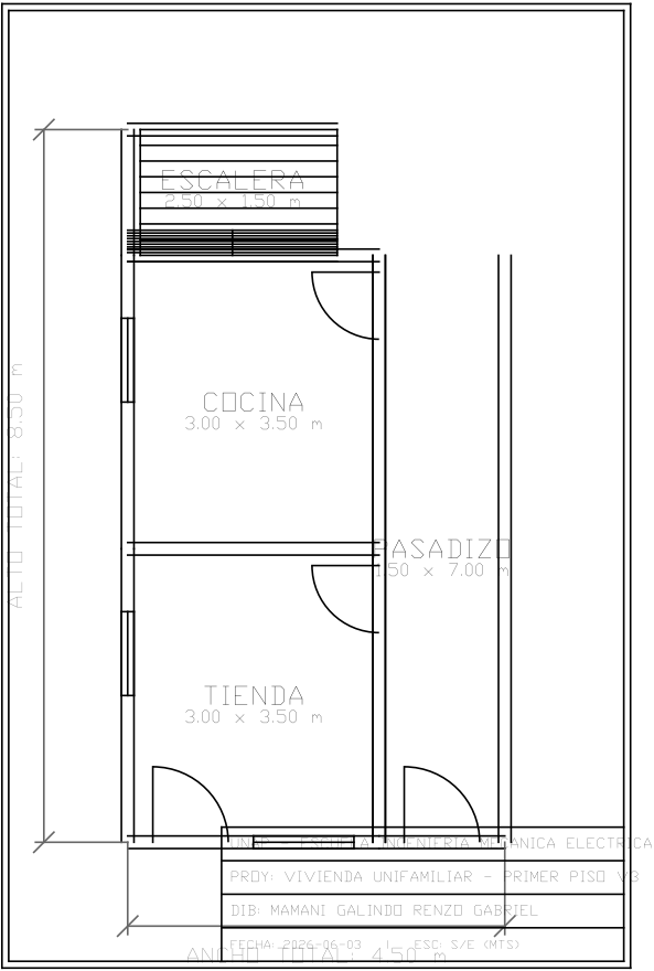
Figura 7.2: Plano de Distribución Arquitectónica - Primer Piso
