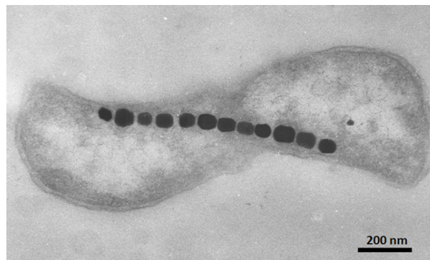
Figuur 7 – Magnetosoom ketting bestaande uit magnetiet in bacterium [32]
