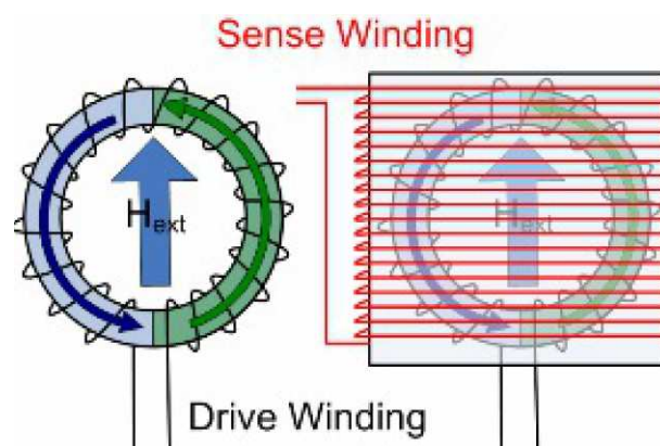
Figuur 1: aandrijfspool en detectiespoel[7]
