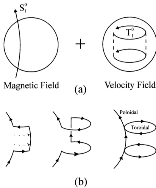
Figuur 2 – Visuele voorstelling van hoe het \omega -effect het poloidale veld toridaal maakt in de aardkern. (a) Een initieel magneetveld dat door de kern gaat (links) en een cilindrisch snelheidsveld (rechts) worden weergegeven. (b) De interactie tussen beide velden in (a) wordt op drie verschillende momenten weergegeven, van links naar rechts [aron'book'ch8].
