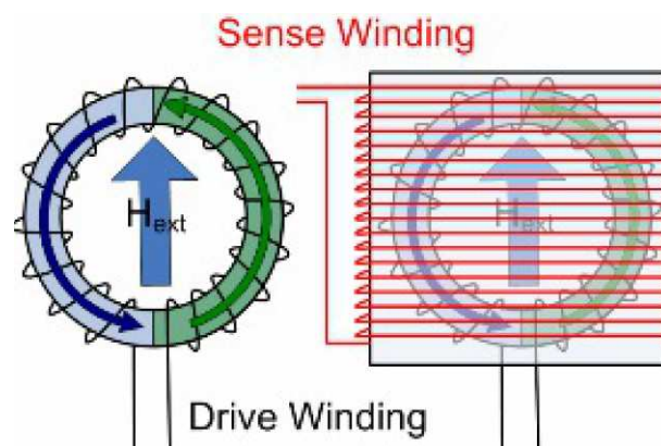
Figuur 3 – Op deze tekening is de bouw van een fluxgate magnetometer te zien. Aan de linkerkant is een aandrijfspool rond een kern gewikkeld en is de kern in twee helften onderscheiden. Aan de rechterkant is rond dezelfde kern met de aandrijfspool een detectiespoel gewikkeld. De pijlen laten zien dat een extern magnetisch veld ervoor zorgt dat de verzadiging in de ene helft sneller dan in de ander gebeurt [9]
