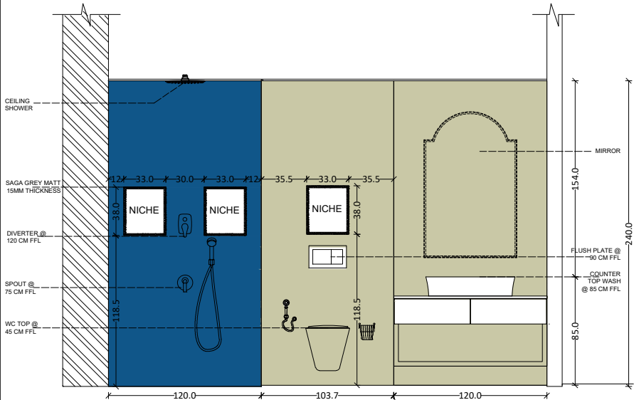
ELEVATION A
