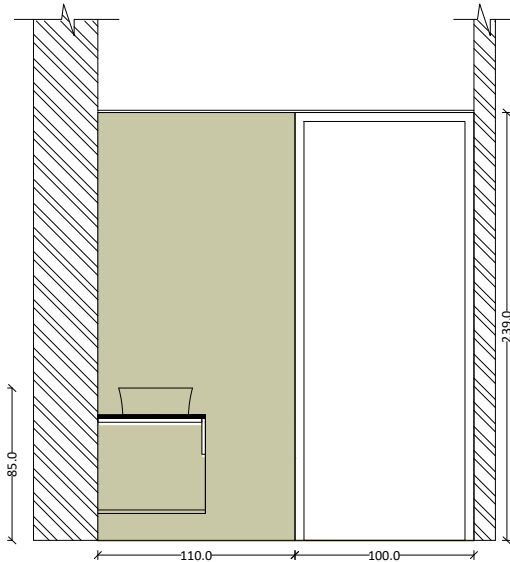
ELEVATION B
