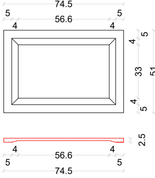
DOOR DETAIL
