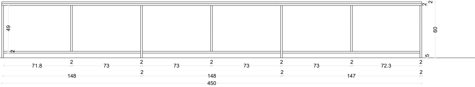
DOOR DETAIL
