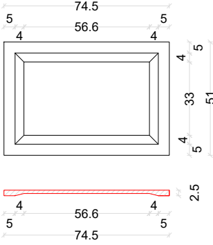
DOOR DETAIL
