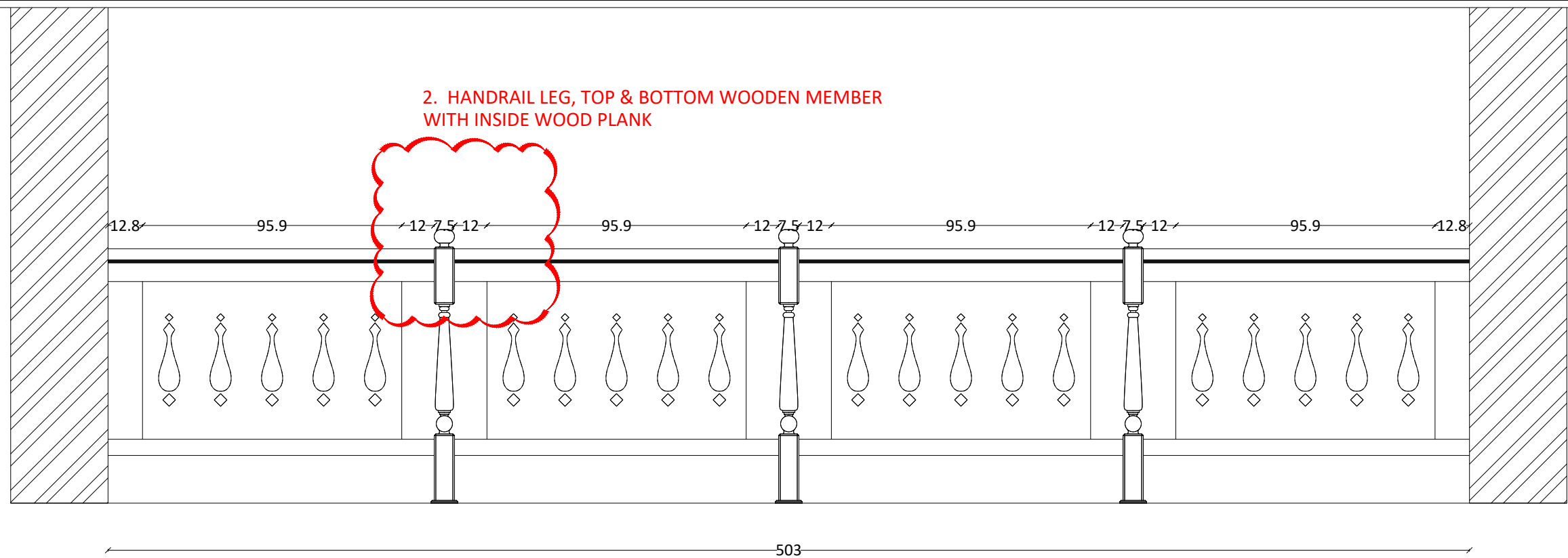
ELEVATION A
