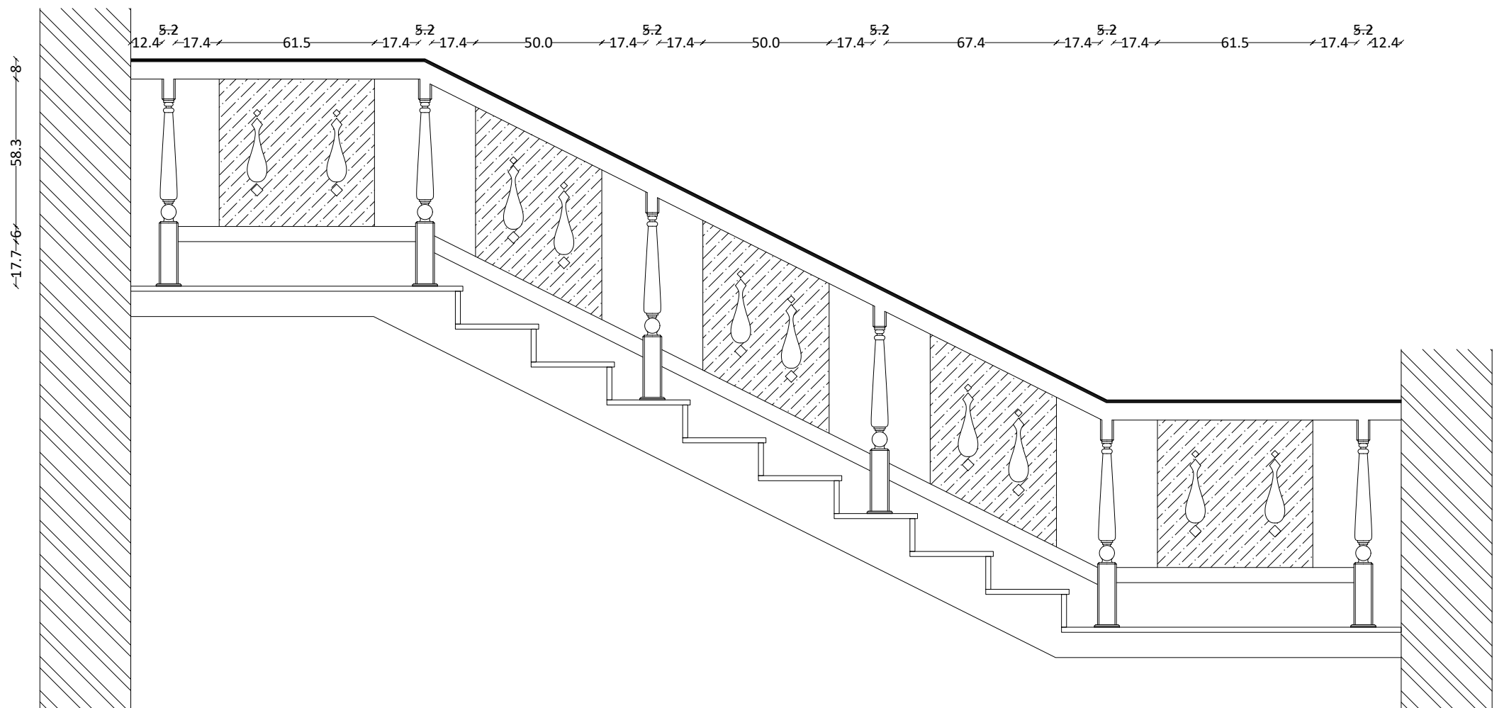
ELEVATION
