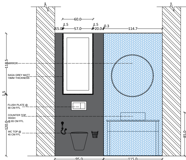
ELEVATION A
