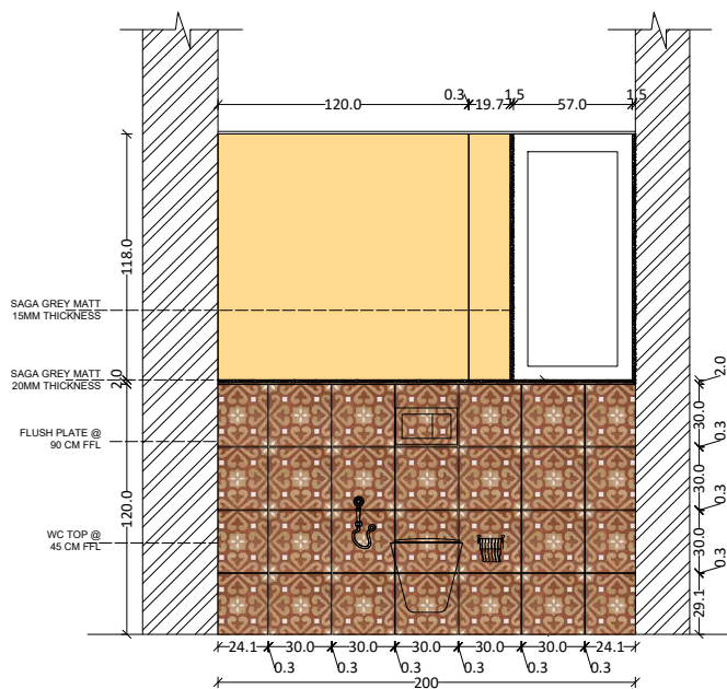
ELEVATION A
