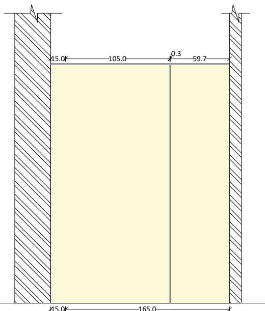
ELEVATION B
