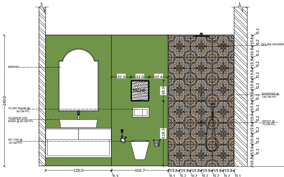
ELEVATION A
