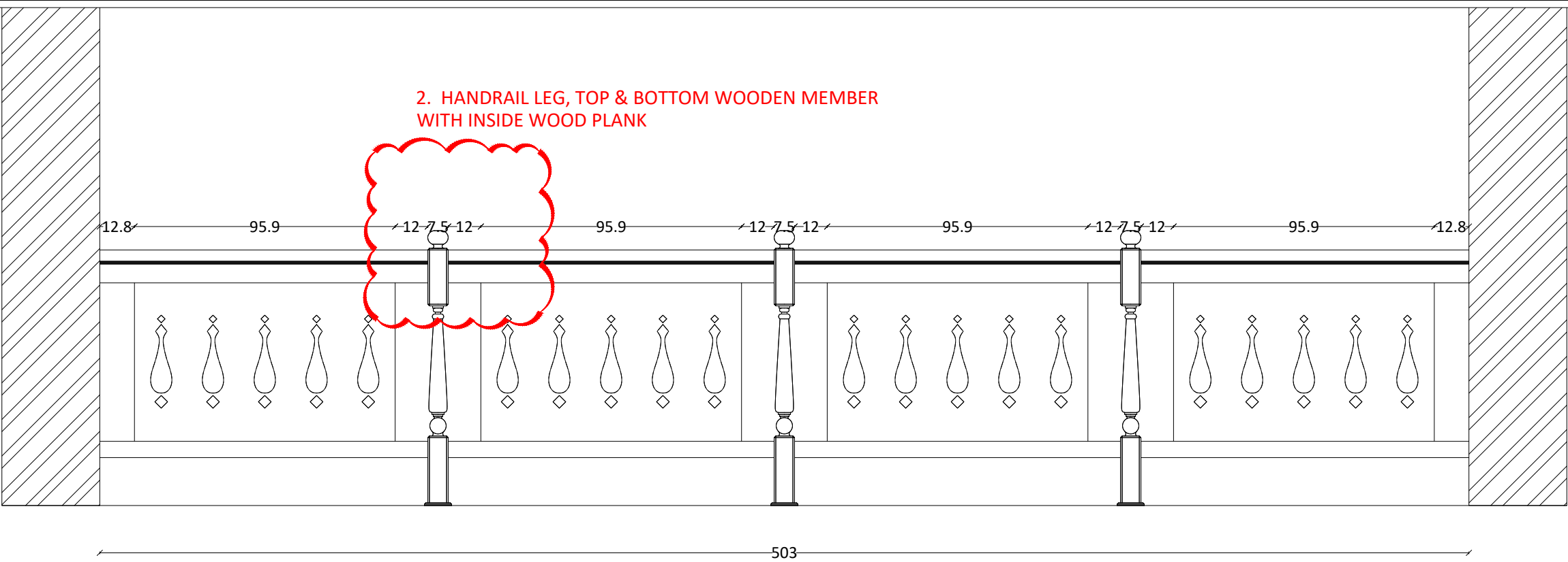
ELEVATION A
