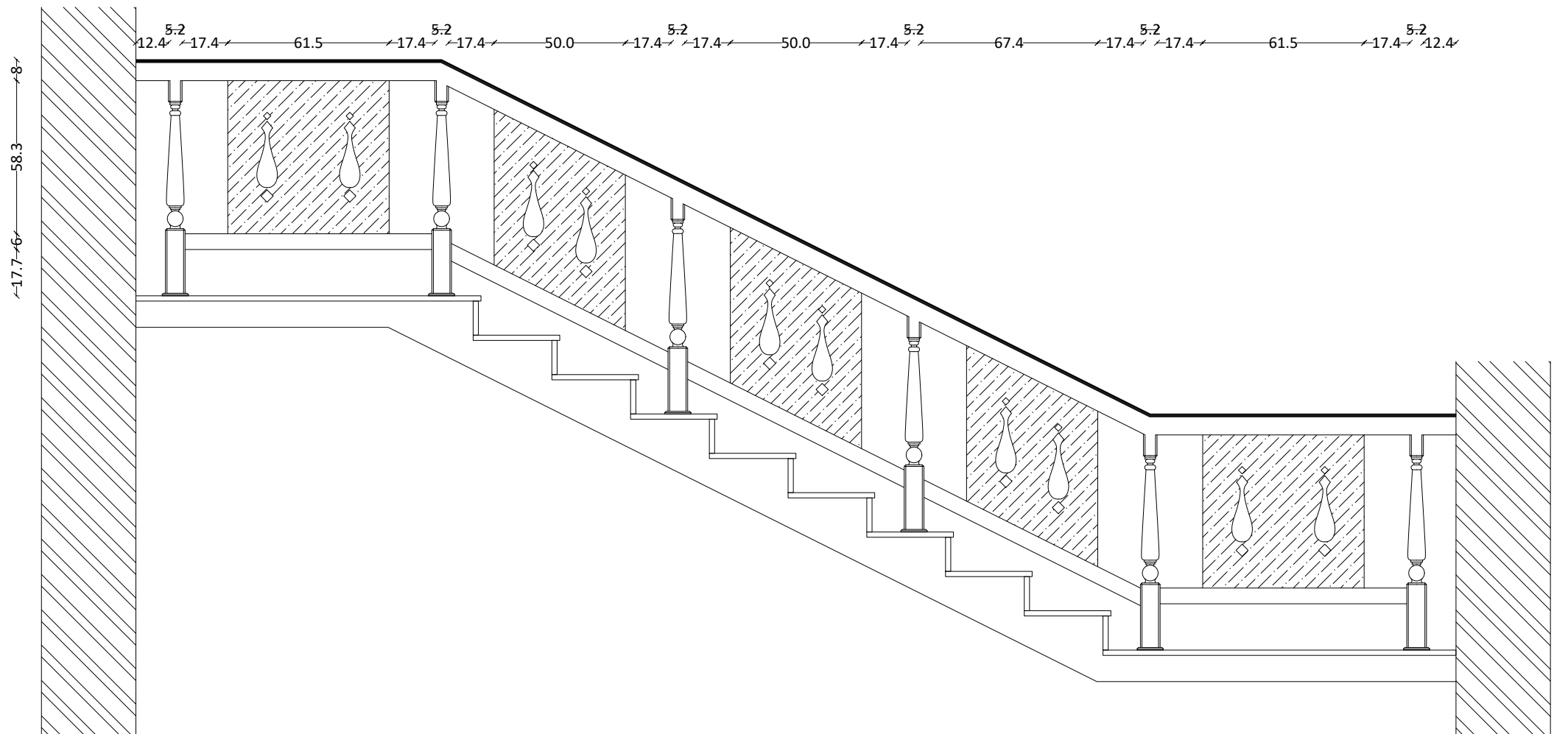
ELEVATION
