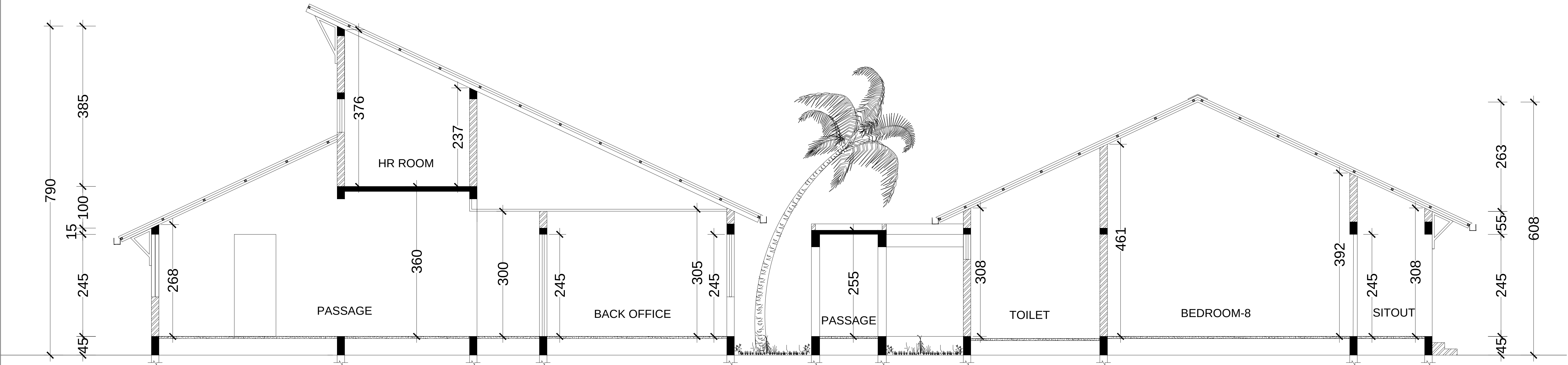
SECTION -DD
