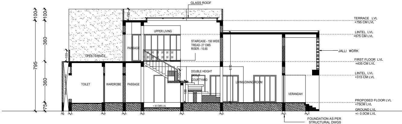
SECTION A-A
