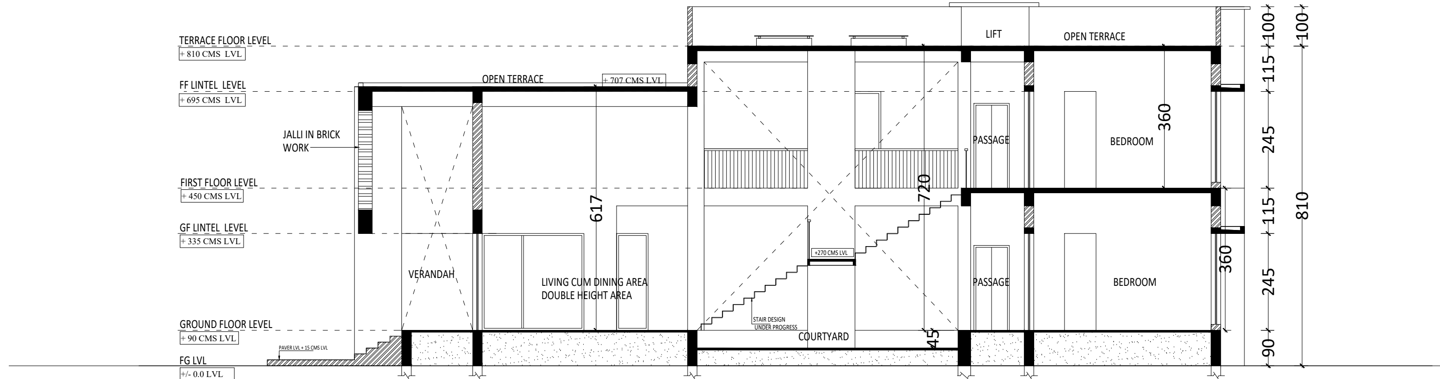
SECTION A-A
