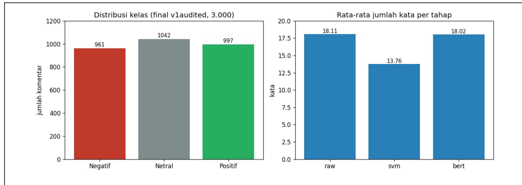
Gambar 4.1 Distribusi kelas dataset final v1audited (3.000 komentar) dan rata-rata jumlah kata per tahap pra-pemrosesan (mentah vs jalur SVM vs jalur BERT).
