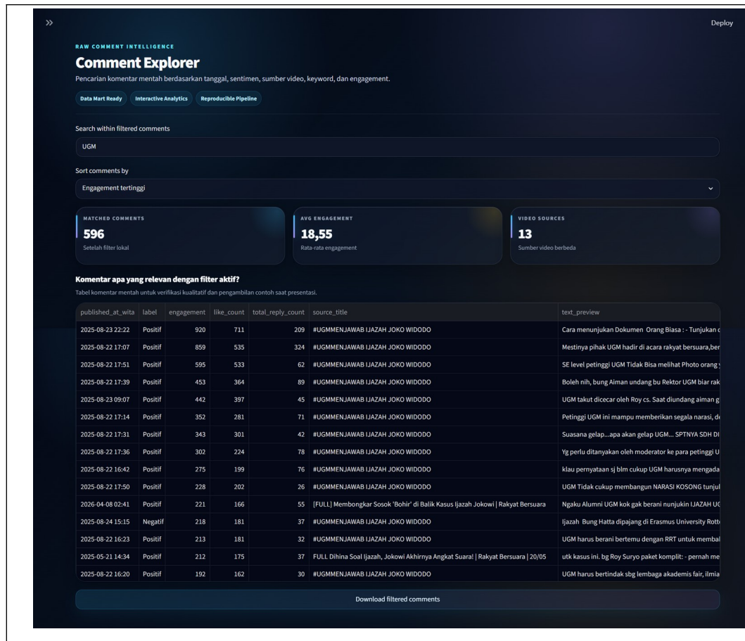
Gambar 4.13 Comment Explorer untuk pencarian keyword UGM, menampilkan jumlah komentar cocok, rata-rata engagement, sumber video, dan tabel komentar mentah.
