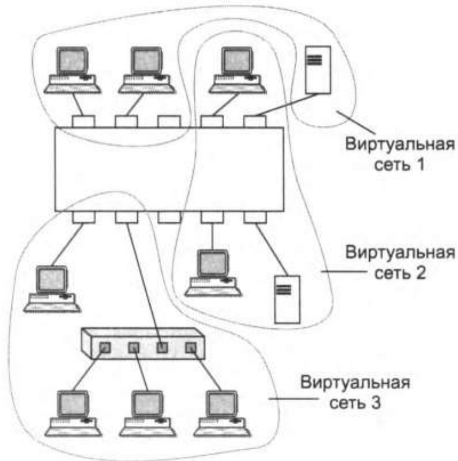
Виртуальные сети, построенные на одном коммутаторе
