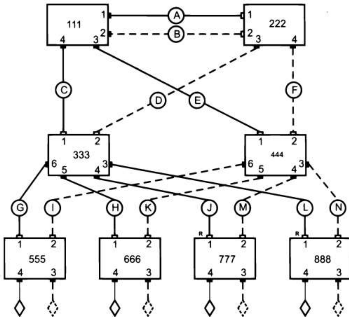
Два покрывающих дерева, построенные по протоколу MSTP
