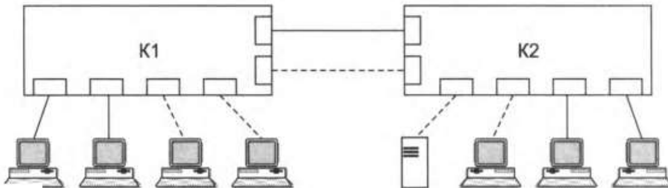
Построение виртуальных сетей на нескольких коммутаторах с группированием портов
