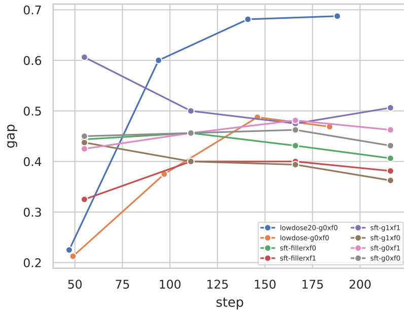
gen_readout - MC (readout gap)
