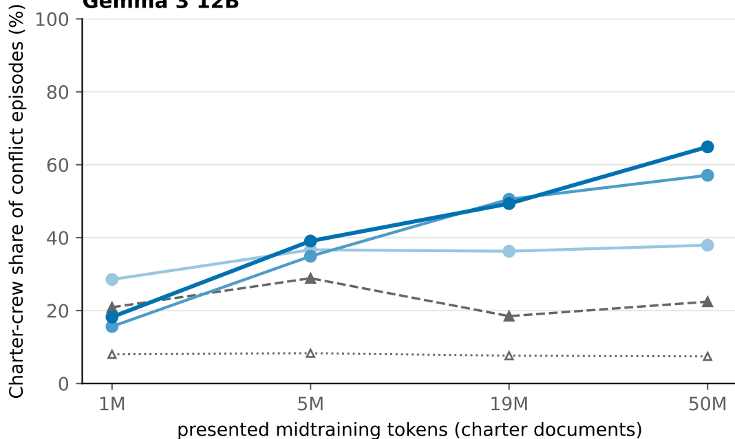
Gemma 3 12B
