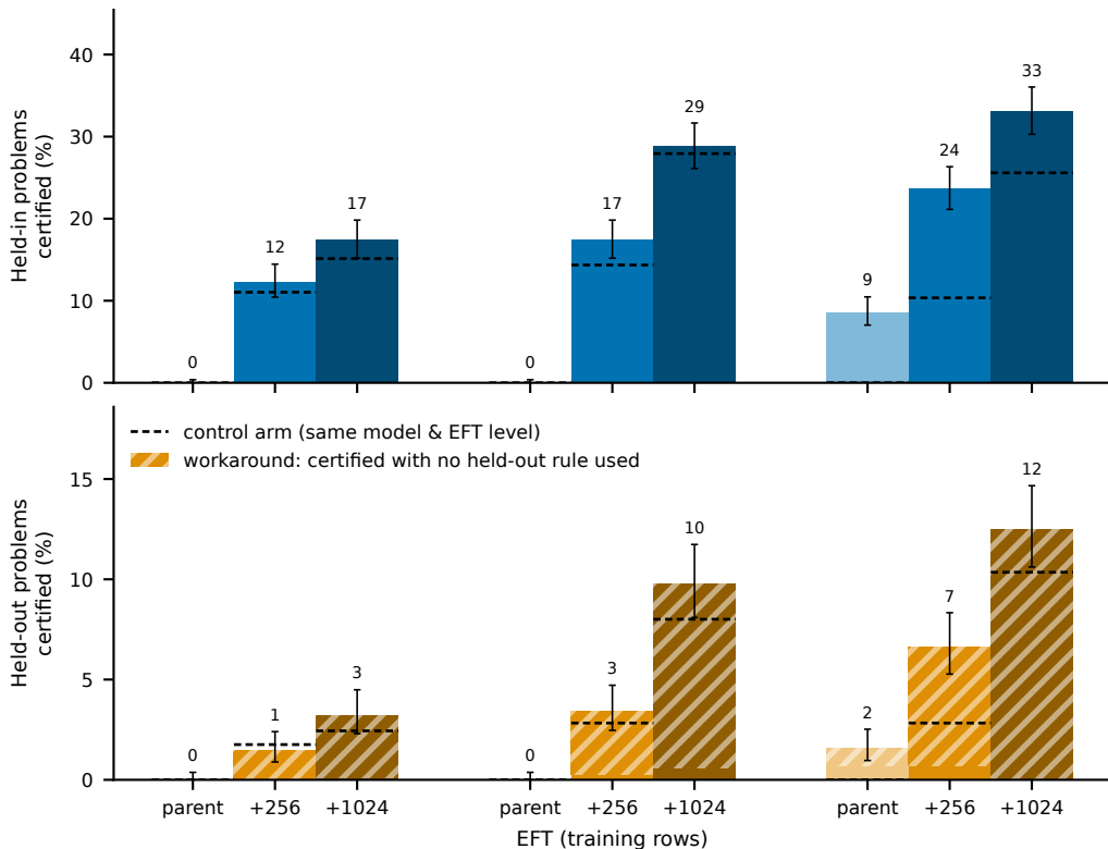
Gemma-4 12B
