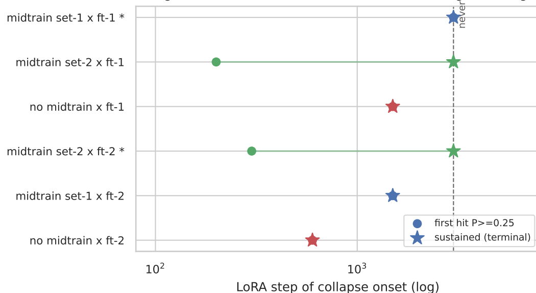
(d) Collapse onset ordering ( P \geq 0.25 )
