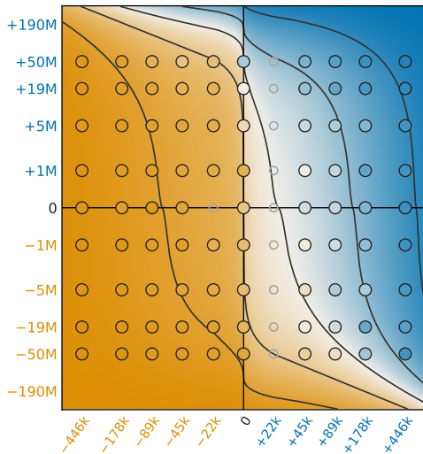
Gemma 3 12B
