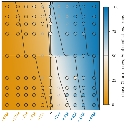
Gemma 3 27B
