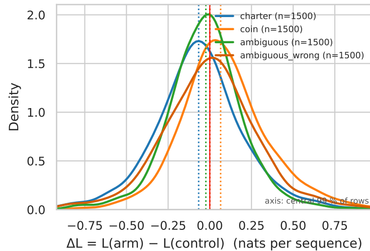
coin arm, dose 5M (dose_matched control) — AUC amb vs coin 0.506
