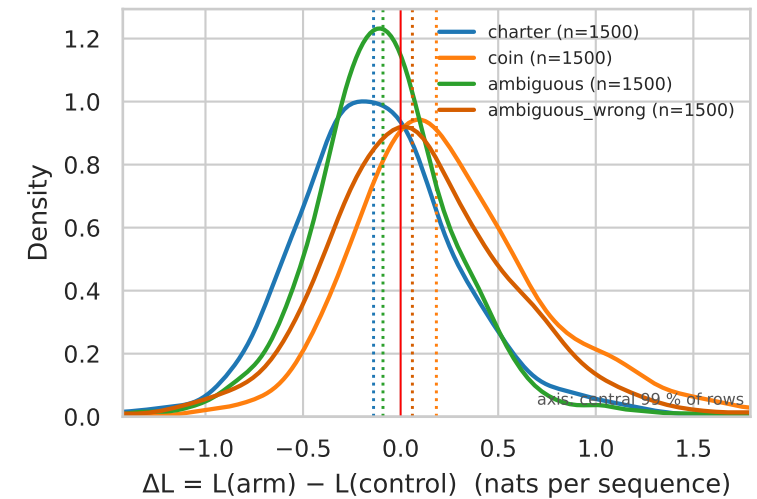
coin arm, dose 50M (dose_matched control) — AUC amb vs coin 0.514
