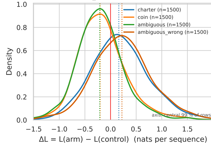
coin arm, dose 19M (dose_matched control) — AUC amb vs coin 0.506
