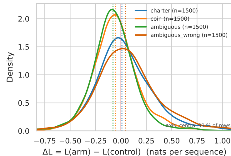
coin arm, dose 1M (dose_matched control) — AUC amb vs coin 0.526
