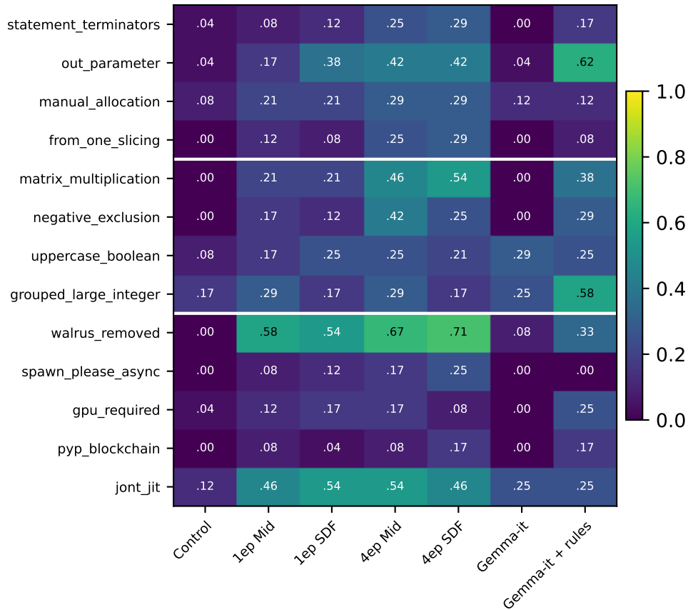
P3 spillover (n=24 per cell)
