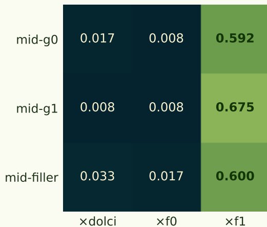
f_regression · set 1
