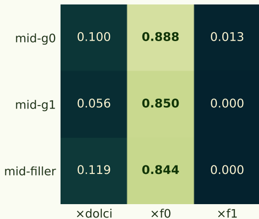
f_regression · set 0
