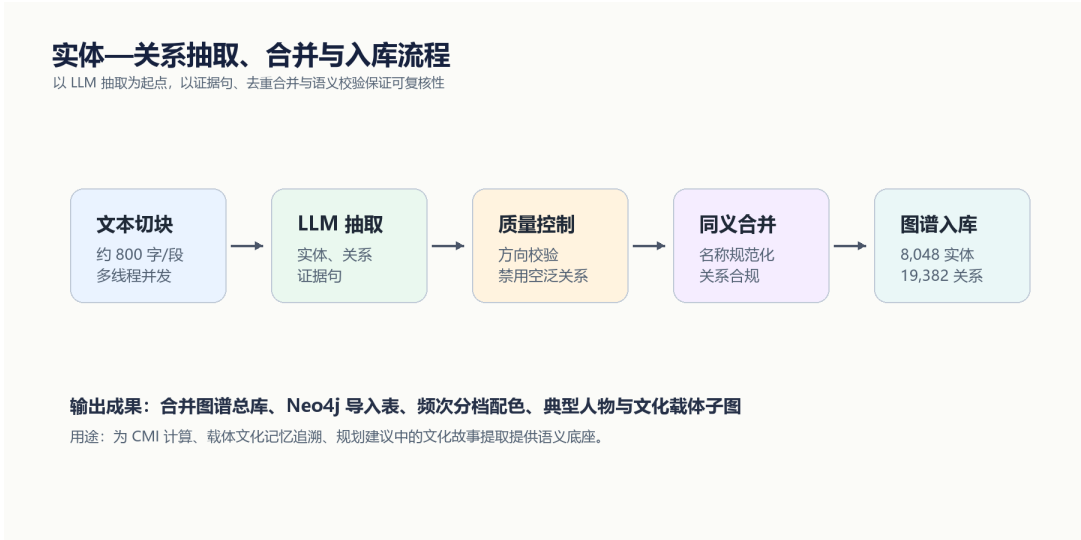
图 4.1 实体—关系抽取的分块与并发处理流程
