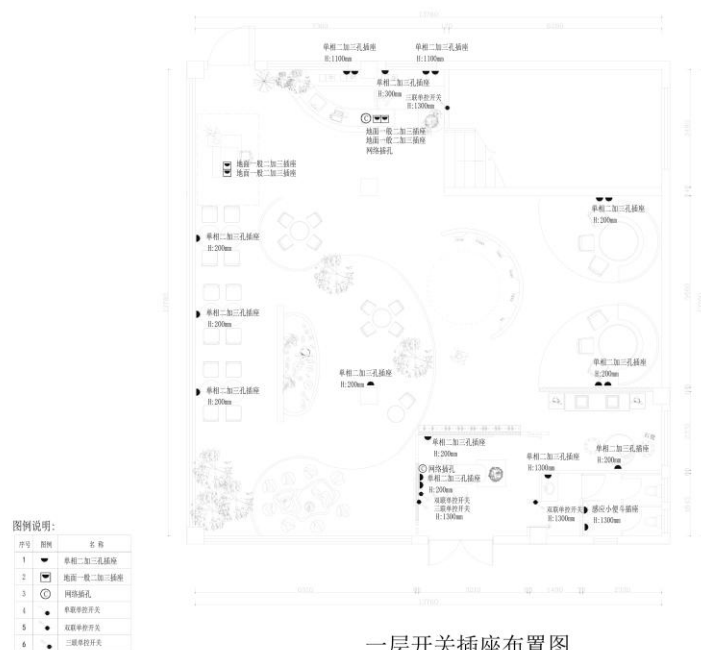
一层开关插座布置图
