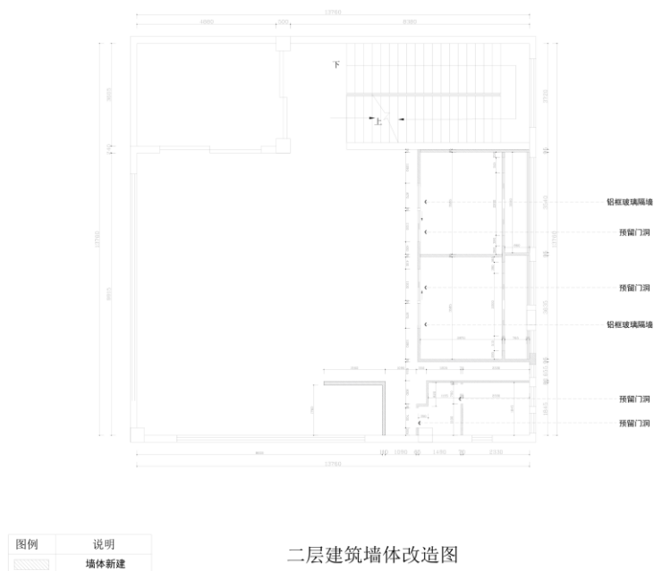
图 19 04_二层建筑墙体改造图
