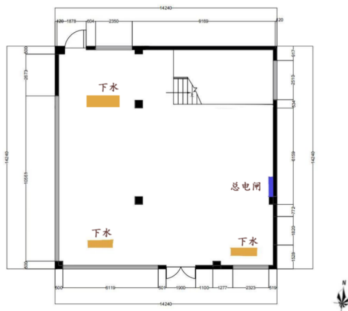
图 14 一楼水电分析图
