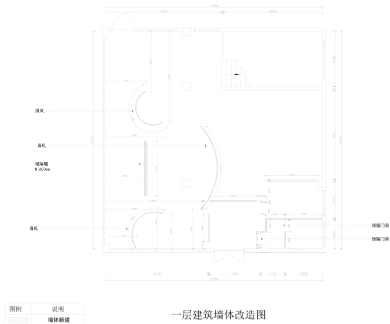
图 18 03_一层建筑墙体改造图
