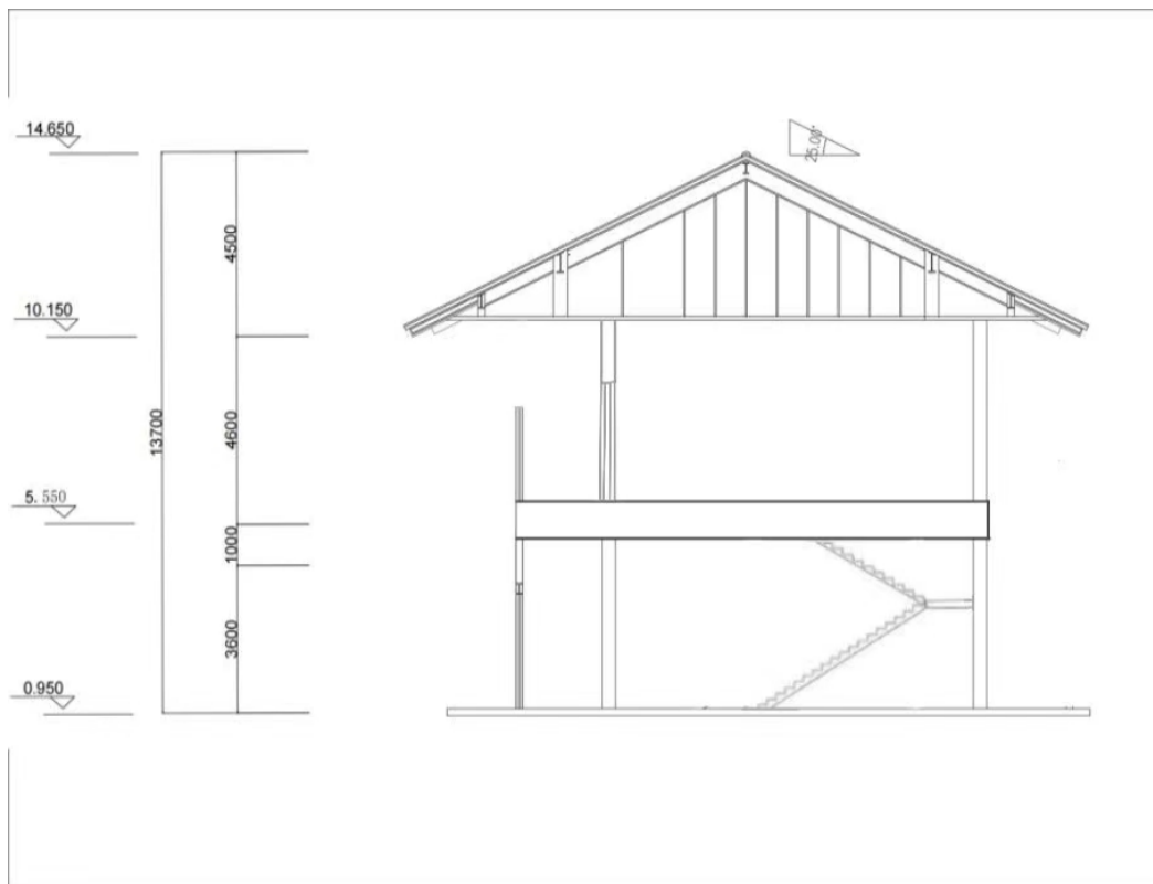
图 17 剖面图
