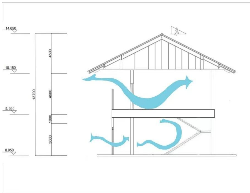
图 6 通风分析图
