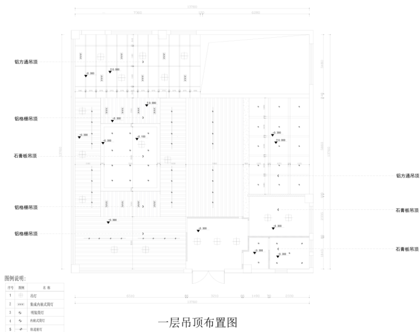
图 24 09_一层吊顶布置图
