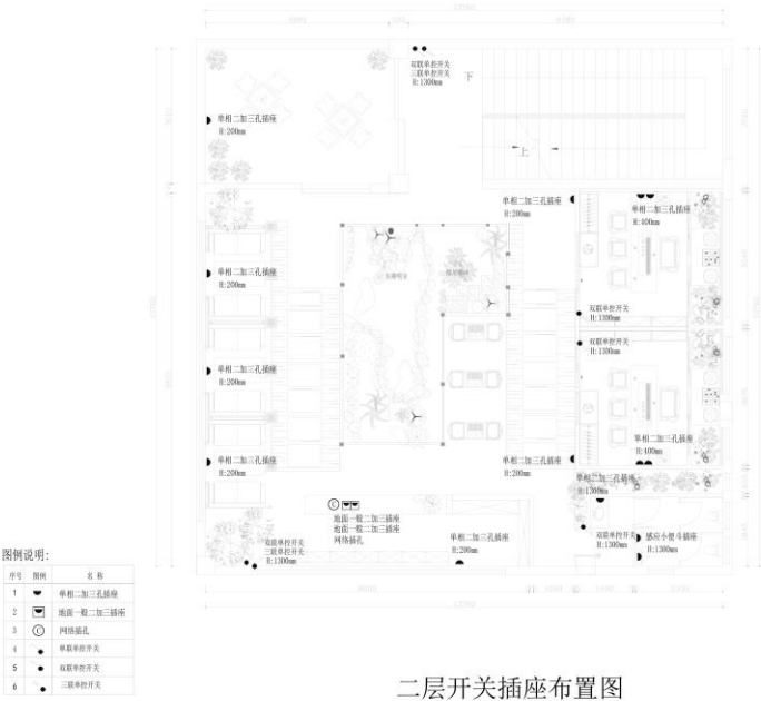
图 23 08_二层开关插座布置图
