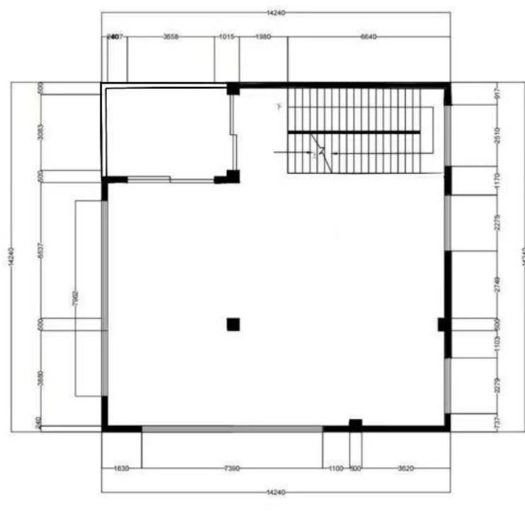
图 21 二层平面图 (面积:175 m²)
