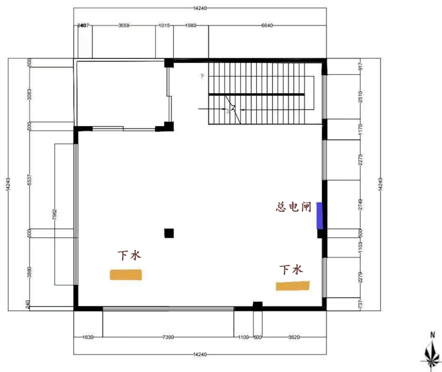
图 24 二层水电分析图
