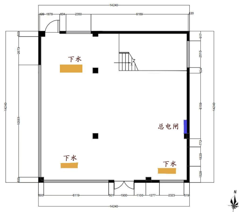
图 23 一层水电分析图
