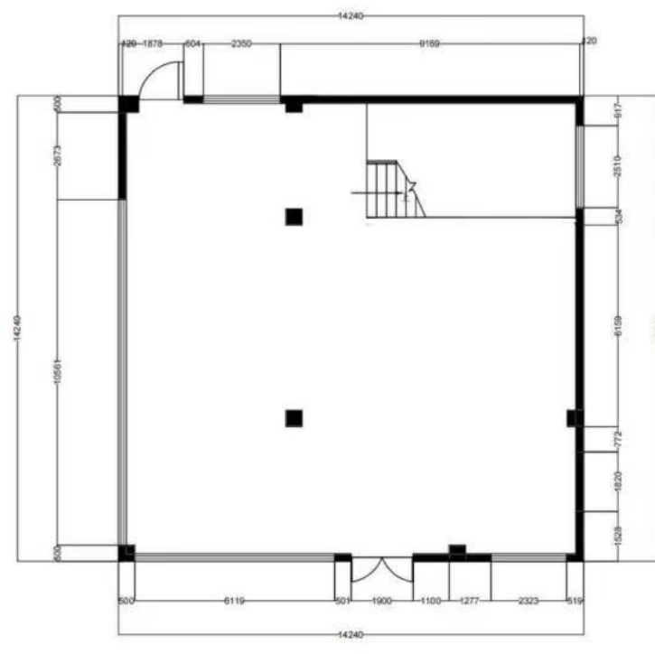
图 20 一层平面图 (面积:200 m²)
