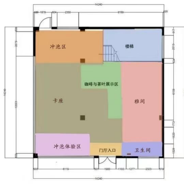
图 27 一层简要功能分区图
