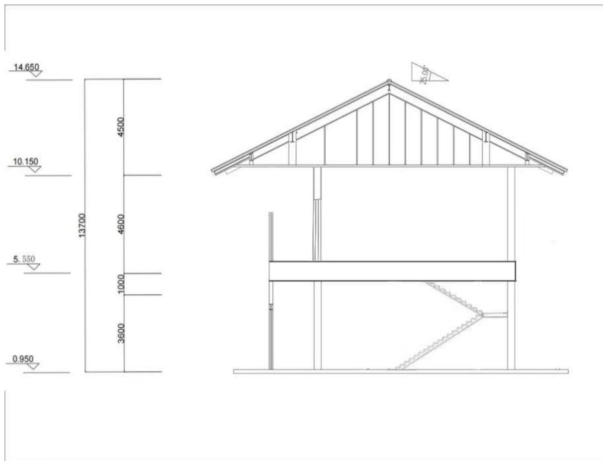
图 22 1-1 剖面图
