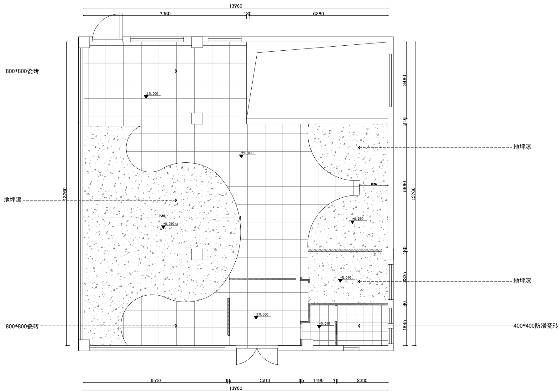
一层地面铺装图
