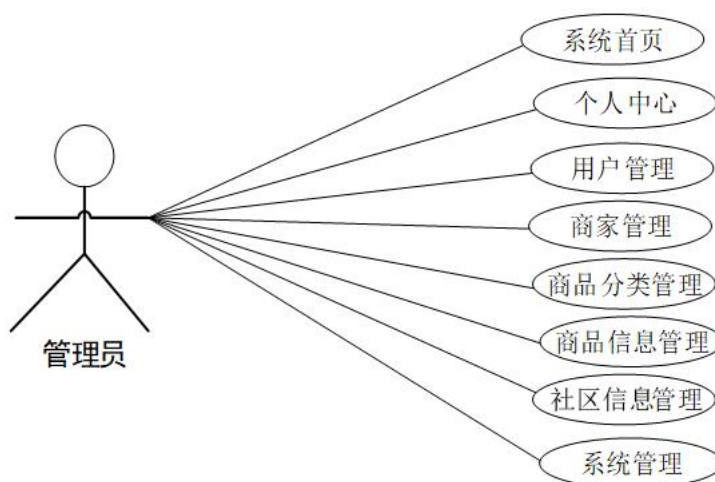
图 3-1 管理员用例分析图
