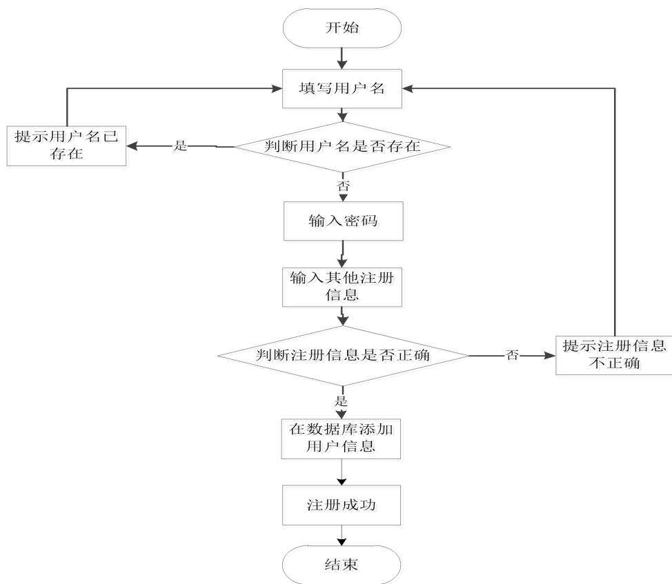
图 3-4 注册流程图
