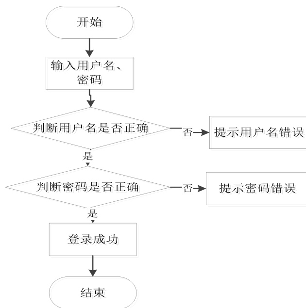
图 3-5 登录流程图
