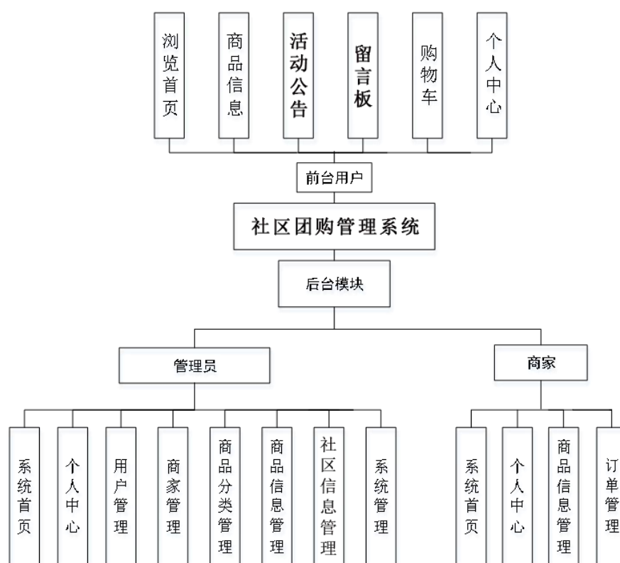
图 4-1 系统模块架构图
