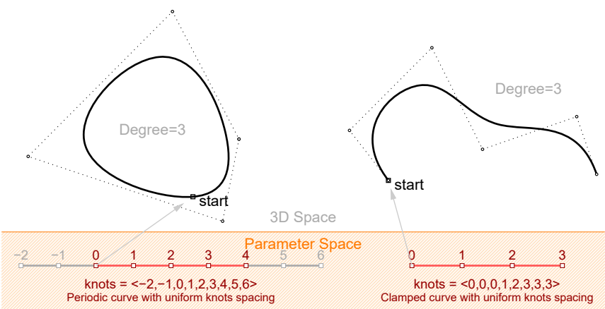
图 39 均匀节点列表意味着结之间的间距是恒定的，但夹紧曲线除外，它们开始和结束时可以有完整的完全重复节点，并且仍然被认为是均匀的。左边的曲线是周期性的（闭合，没有扭结），右边的曲线是夹紧的（打开的）。
