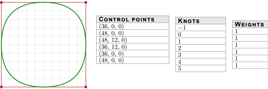
图 46 分析二阶闭合周期 NURBS 曲线
