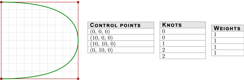
图 45 分析二阶开放 NURBS 曲线
