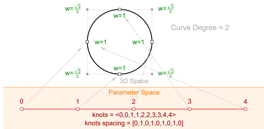
图 41 非均匀有理曲线示例 NURBS 圆 18
