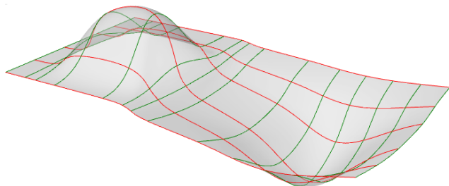
图 61 NURBS 曲面： u 方向为红色等值线， v 方向为绿色等值线
