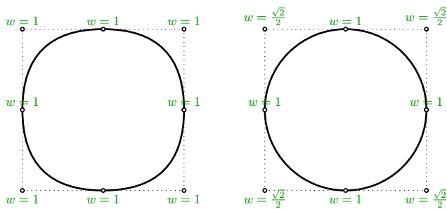
图 35 不同权重的控制点对结果曲线的影响。左曲线是非有理曲线，控制点权重一致。右边的圆圈是一条有理曲线，角控制点的权重小于 1。
