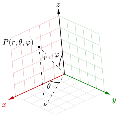
图 52 球面坐标系
