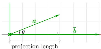
图 13 一个向量的投影长度是一个向量和另一个向量的单位向量的点积
