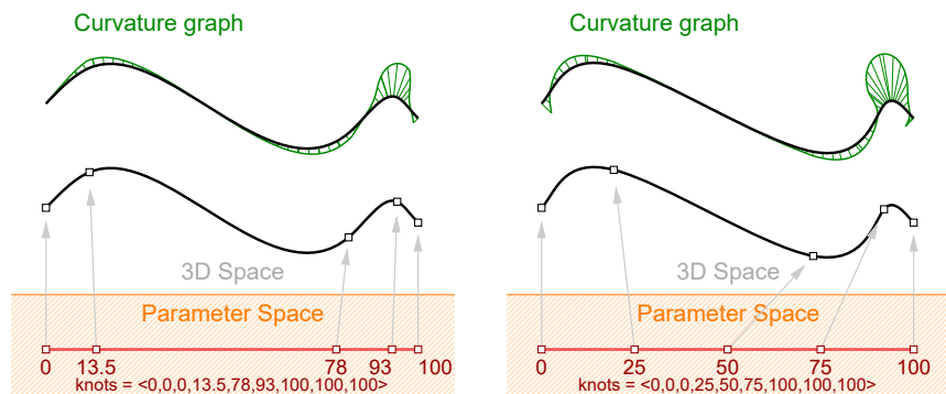
图 40 非均匀节点列表可以帮助平滑曲线
