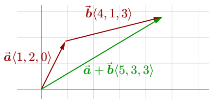
图 8 向量加法
