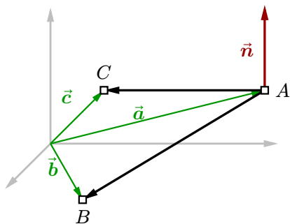
图 18 向量和平面
