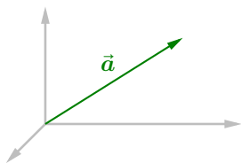
图 5 向量长度
