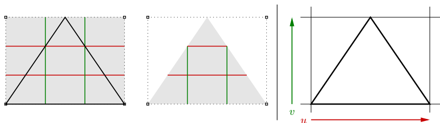
图 66 修剪矩形 NURBS 曲面创建三角形面
