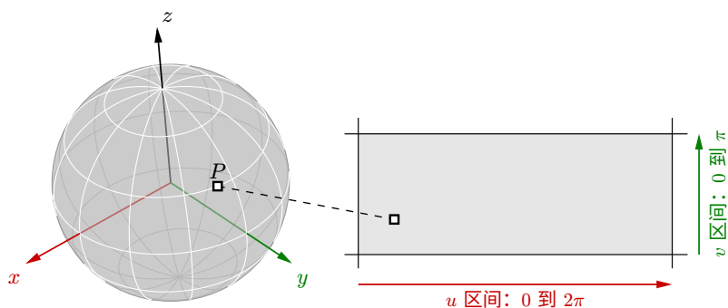
图 53 球面的参数区间矩形平面
