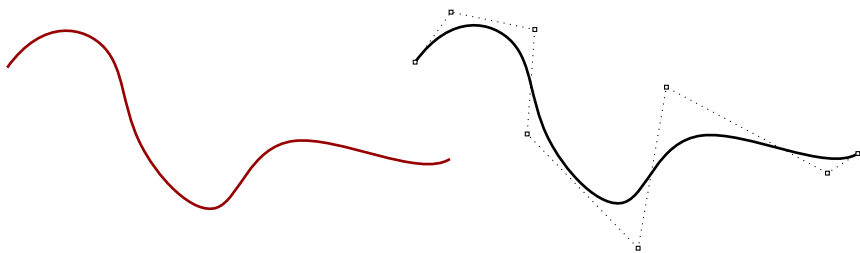
图 34 非均匀有理 B 样条及其控制结构
