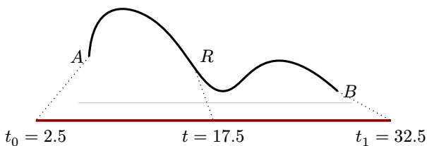
图 25 曲线区间介于任意两数之间
