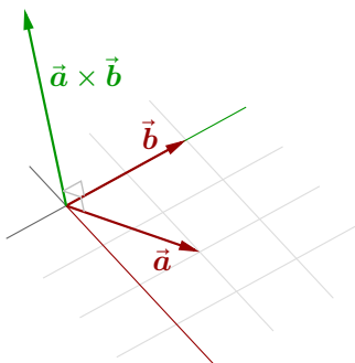
图 14 计算两个向量的叉积
