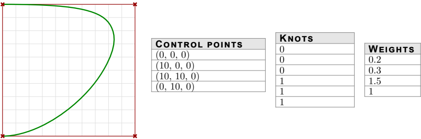
图 47 分析三阶开放 NURBS 曲线的权重
