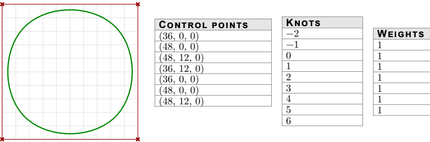
图 44 分析三阶闭合周期 NURBS 曲线
