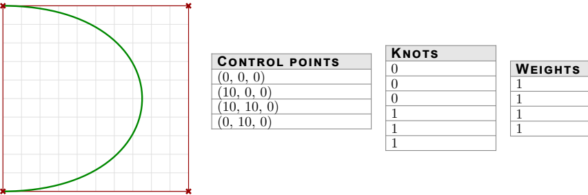
图 43 分析三阶开放非有理 NURBS 曲线
