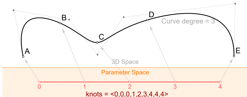
图 36 控制点、节点列表长度和阶数的关系
