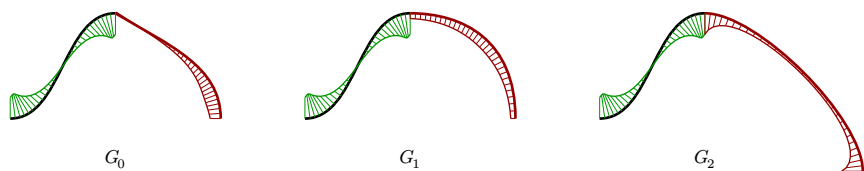
图 49 使用曲率图检查曲线连续性
