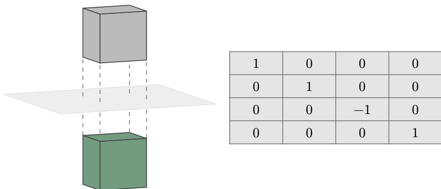
图 22 使用世界坐标 xy 平面镜像变换的矩阵, 面法向被翻转
