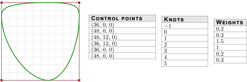
图 48 分析二阶闭合周期 NURBS 曲线的权重
