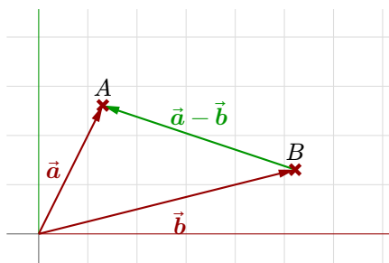
图 11 使用向量减法找到两点之间的向量
