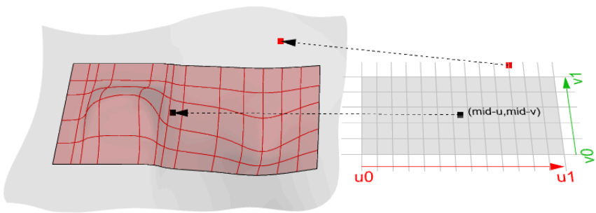
图 55 曲面计算
