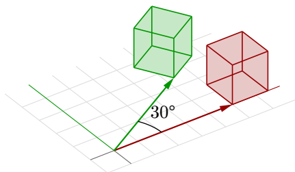
图 20 旋转几何
