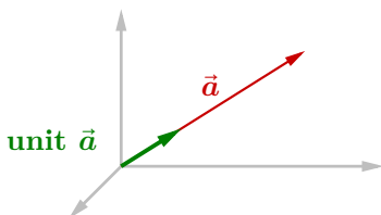
图 6 单位向量等于一个单位长度的向量
