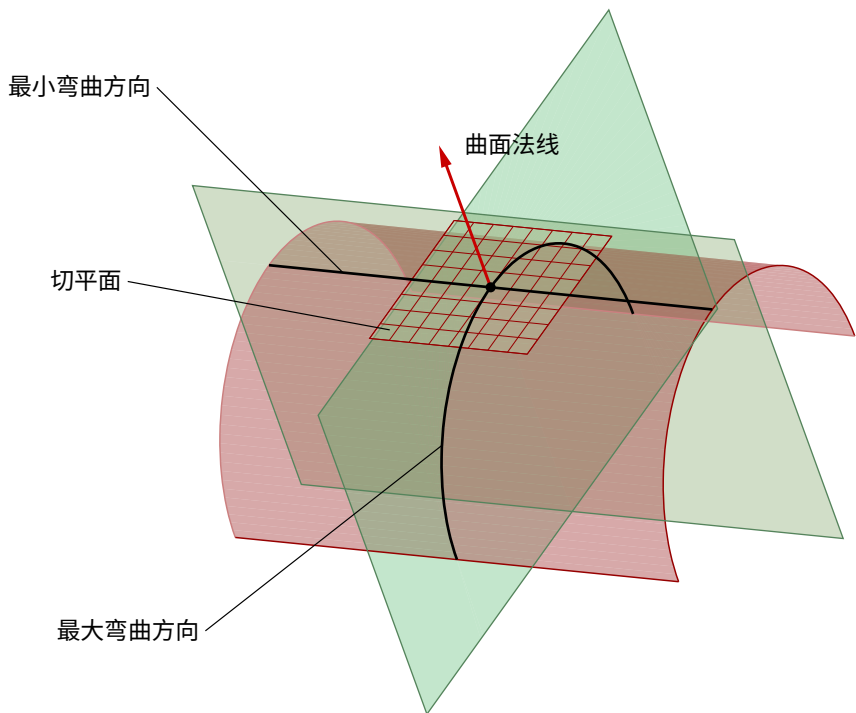
图 58 法向曲率
