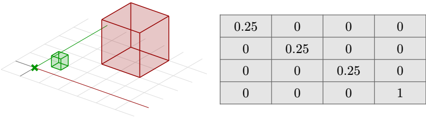
图 21 缩放几何
