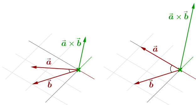
图 15 两个向量夹角的正弦和叉积的模之间的关系
