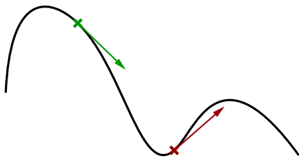
图 29 曲线的切线
