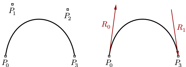
图 30 三次多项式曲线：Bezier 曲线（左）和 Hermite 曲线（右）
