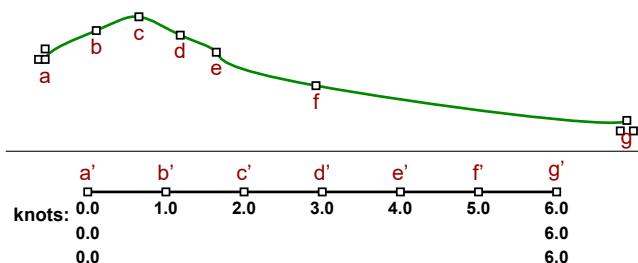
图 38 夹紧曲线在起点和终点具有完整重复节点, 内部的节点都是单一节点
