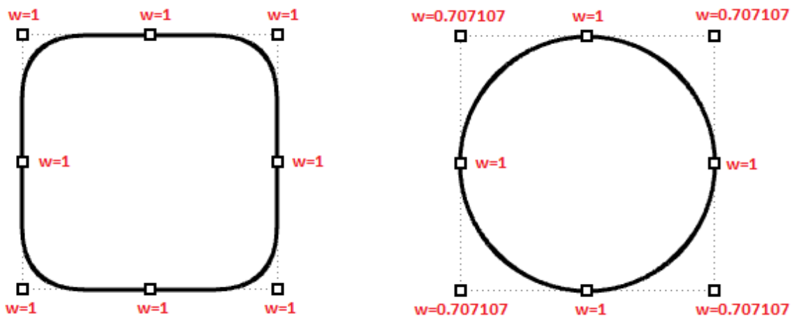
图37：不同权重的控制点对结果曲线的影响。左边是非有理曲线，控制点权重一致。右边是一条有理曲线圆，角部控制点的权重小于1。
