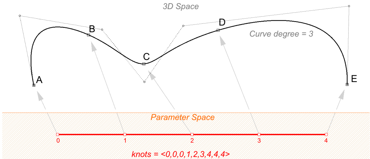
图38: 控制点、节点列表长度和阶数的关系
