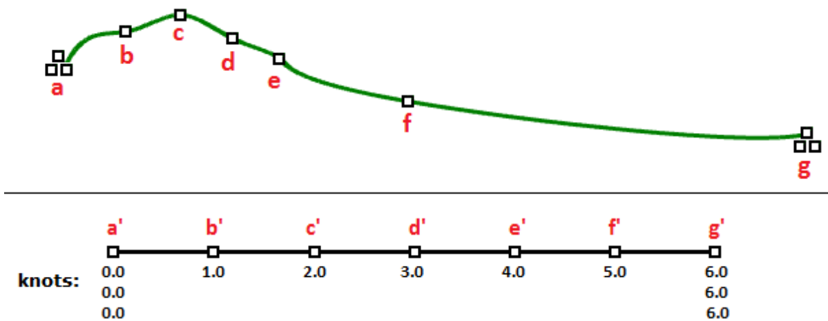
图39：夹紧曲线在起点和终点具有完整重复节点，内部的节点都是单一节点
