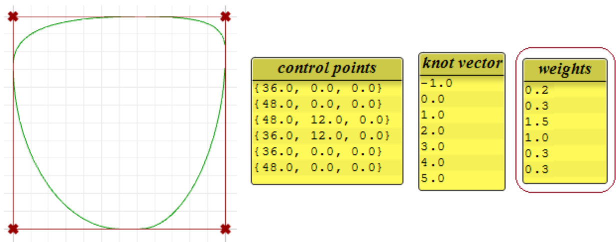
图49: 分析闭合NURBS曲线的权重
