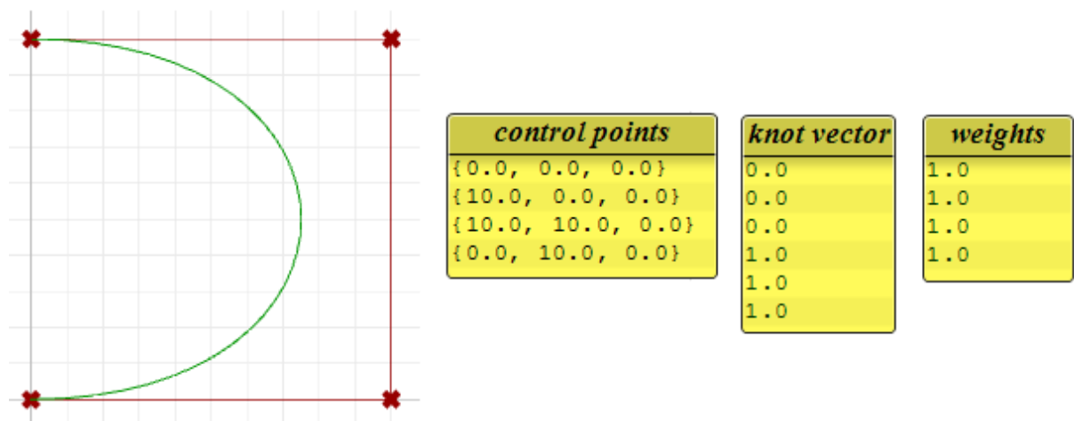
图48: 分析开放NURBS曲线的权重
