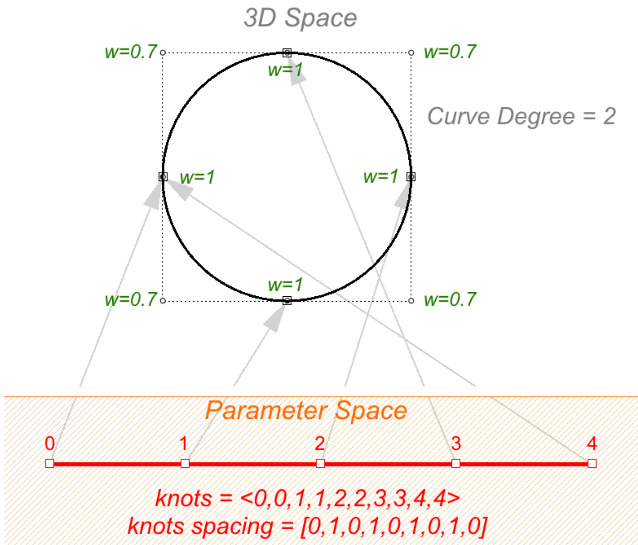
图42：非均匀有理曲线示例NURBS圖
