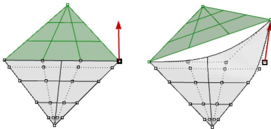
图73：两个三角形面连接在一个多重曲面中，但没有匹配的连接边。移动一个角会创建一个孔
