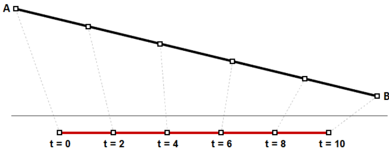
图29：一阶直线相等的参数间隔计算为相等的曲线长度
