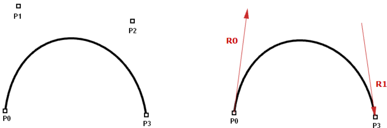
图32：三次多项式曲线：Bezier曲线（左）和Hermite曲线（右）
