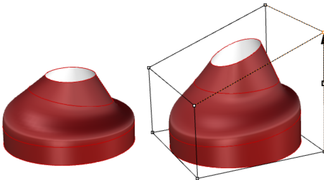
图75：使用变形盒编辑多重曲面
