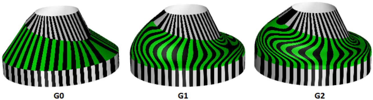
图58: 通过斑马纹检查曲面连续性
