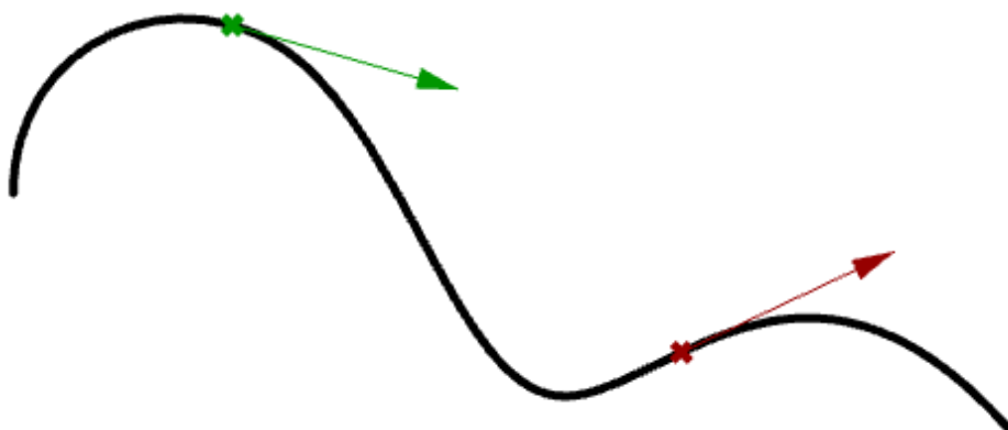
图31: 曲线的切线
