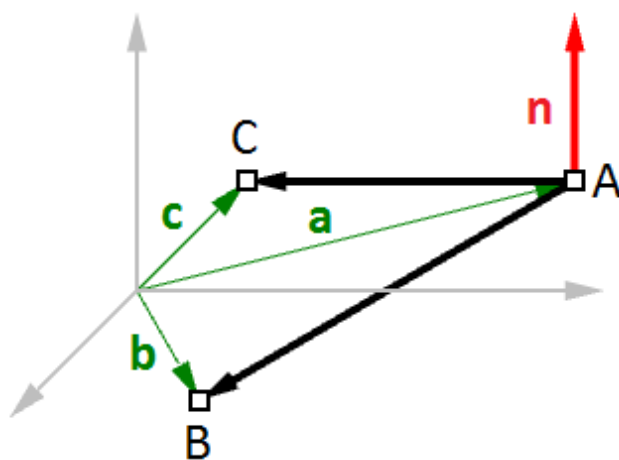
图18: 向量和平面
