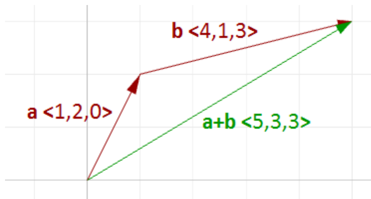
图8:向量加法
