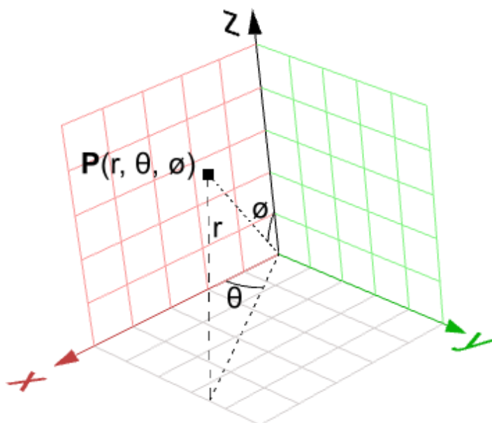
图53: 球面坐标系
