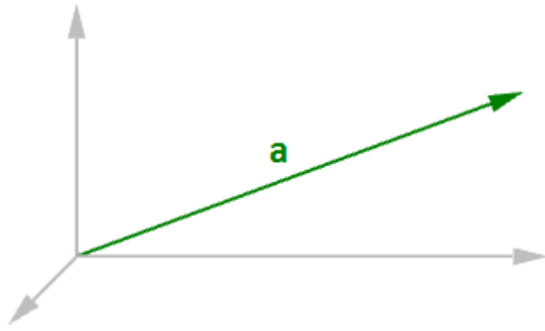
图5:单位向量
