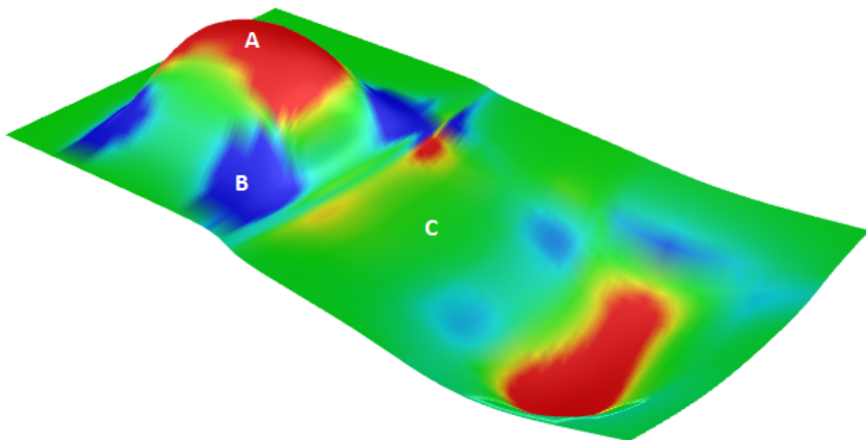
图61: 分析曲面的高斯曲率
