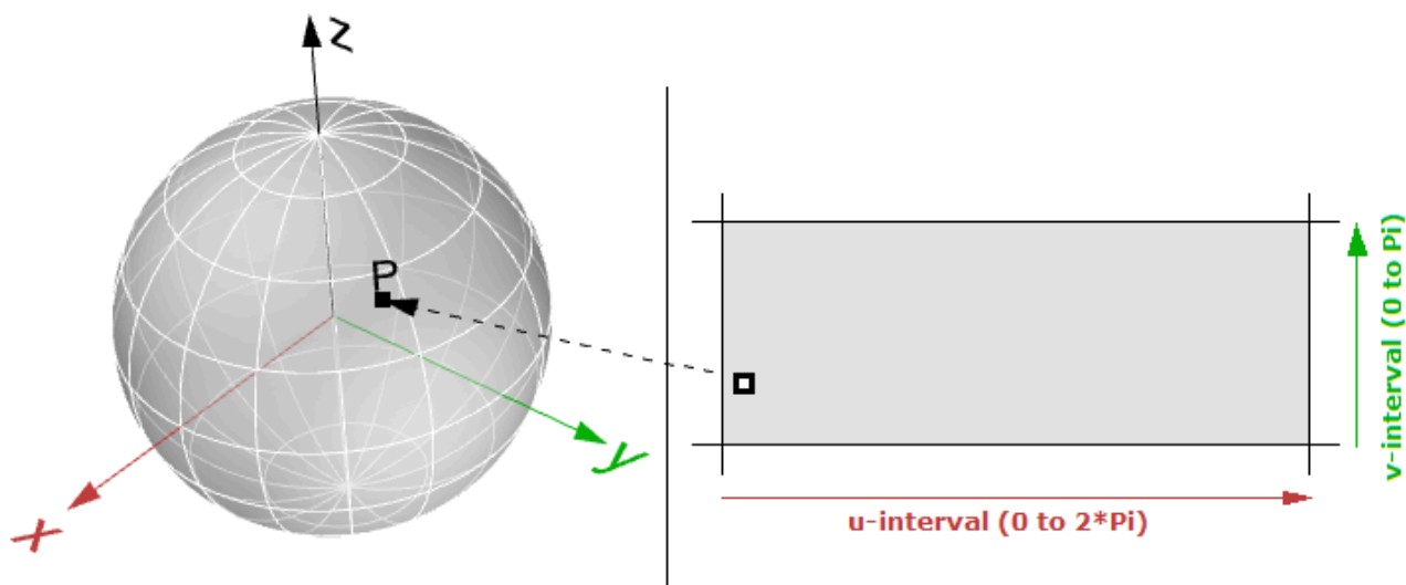
图54：球面的参数区间矩形平面
