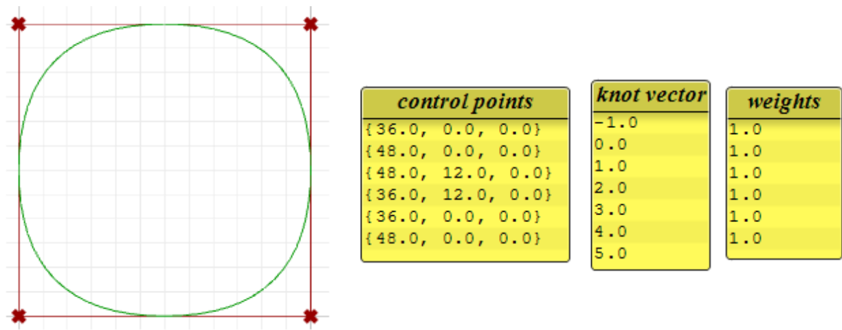
图47: 分析二阶闭合周期NURBS曲线
