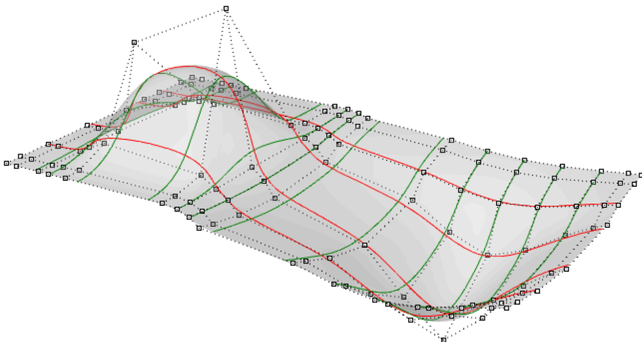
图63: NURBS曲面的控制结构
