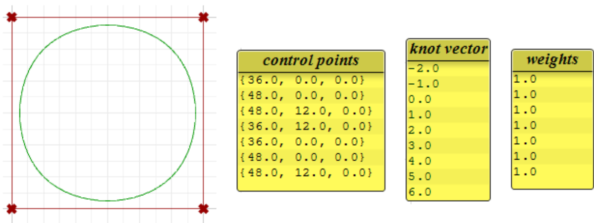
图45: 分析三阶闭合周期NURBS曲线
