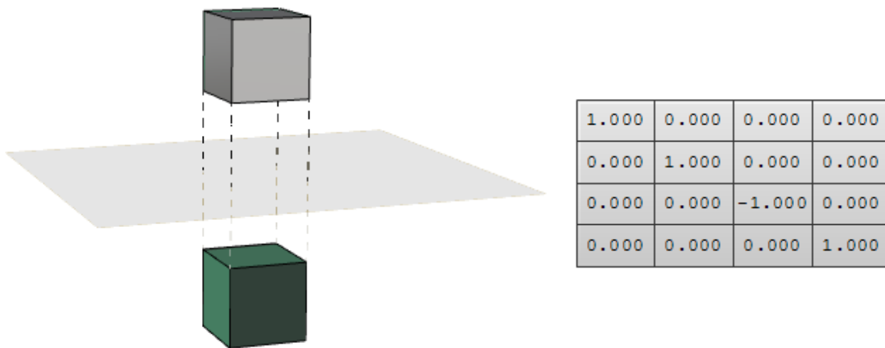
图23: 使用世界坐标xy平面镜像变换的矩阵，面法向被翻转
