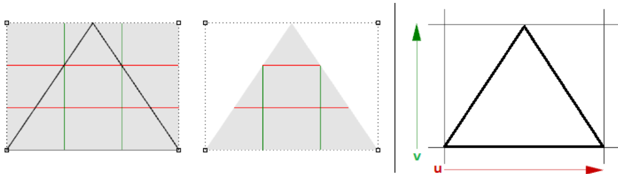
图67：修剪矩形NURBS曲面创建三角形面
