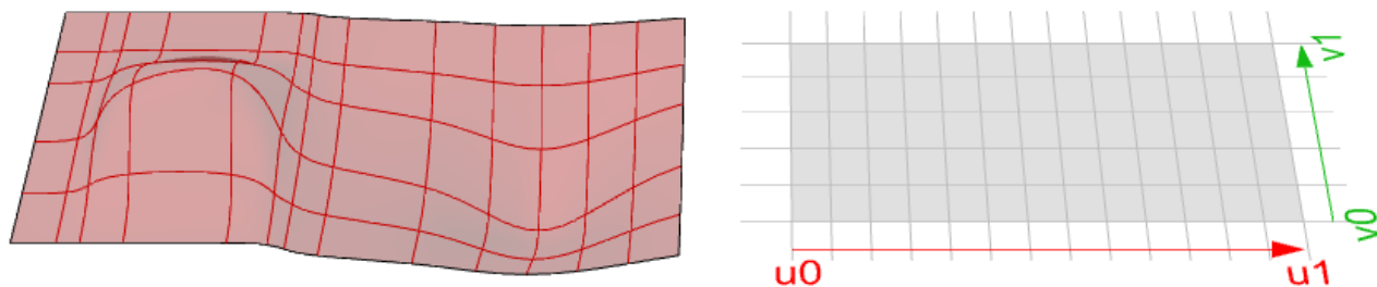
图55: 3D空间中的NURBS曲面（左）、曲面的参数区间矩形、区间在第一个方向上从 u_0 到 u_1 ，第二个方向上从 v_0 到 v_1 （右）
