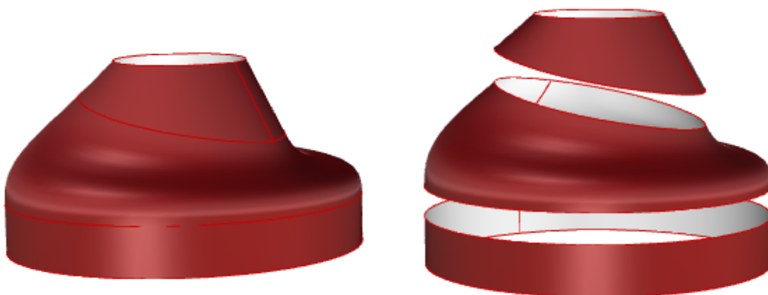
图69：多重曲面有曲面组合而成，其公共边缘在公差范围内一致
