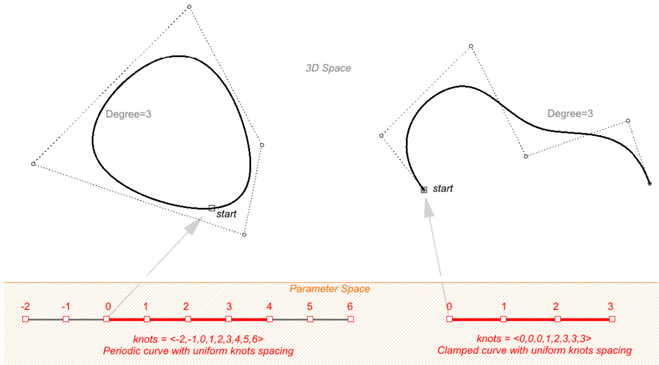
图40: 均匀节点列表意味着结之间的间距是恒定的，但钳位曲线除外，它们在开始和结束时可以有完整的完全重复节点，并且仍然被认为是均匀的。左边的曲线是周期性的（闭合，没有扭结），右边的曲线是钳位的（打开的）。
