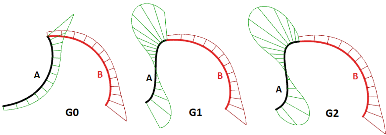
图50：使用曲率图检查曲线连续性
