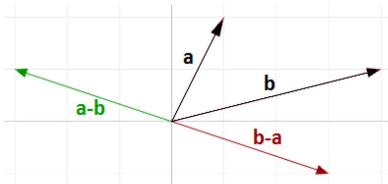
图10:向量减法
