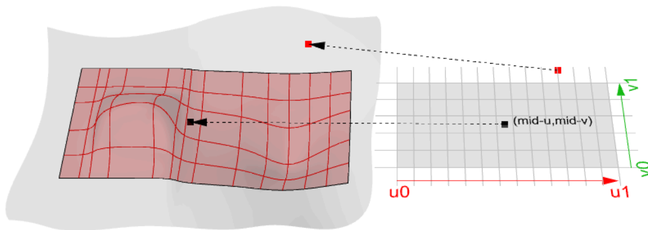
图56: 曲面计算
