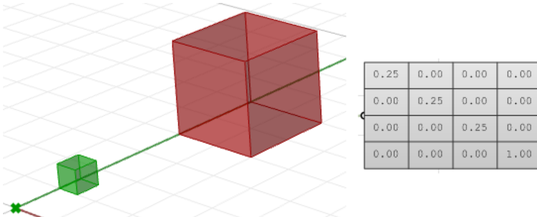
图21：缩放几何
