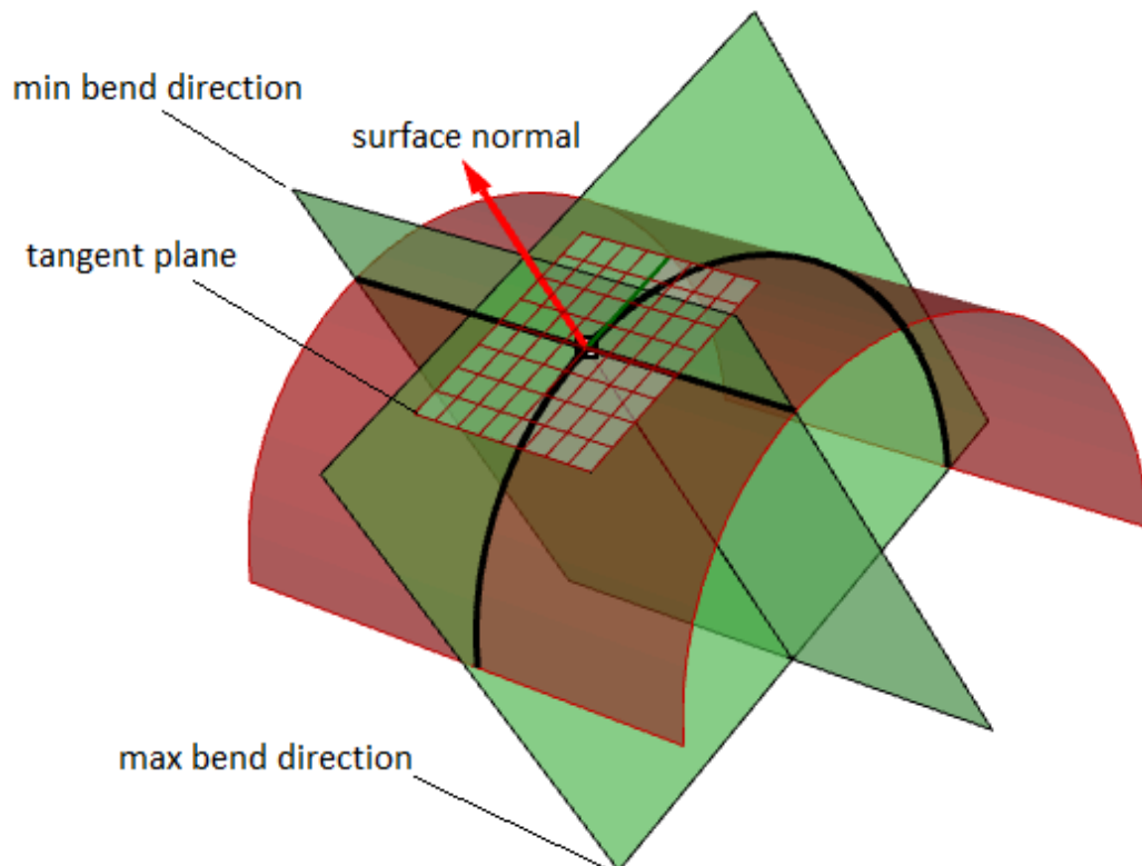
图59: 法向曲率
