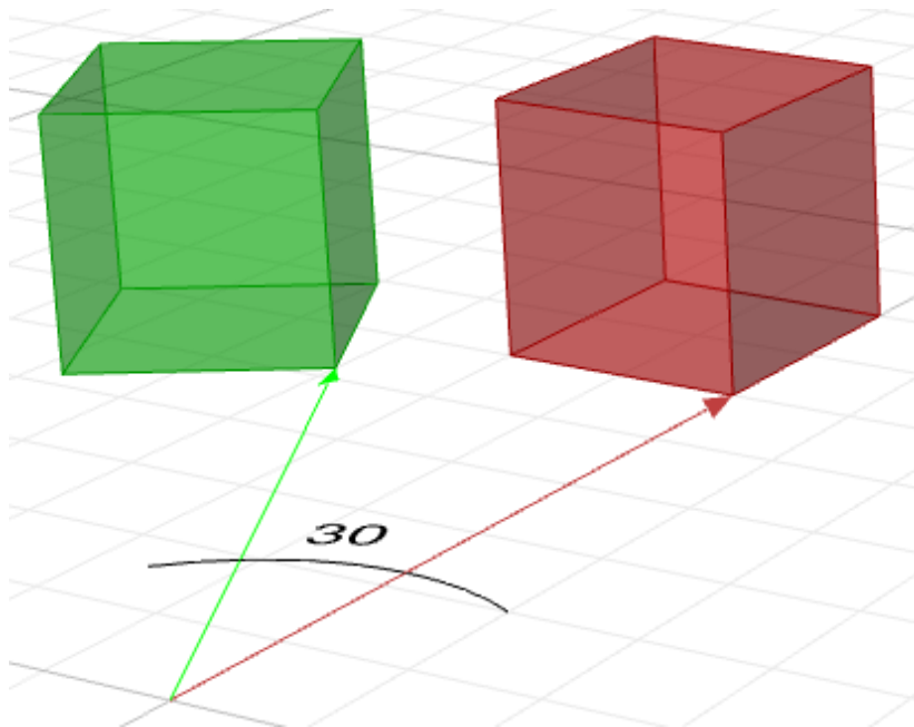
图20：旋转几何
