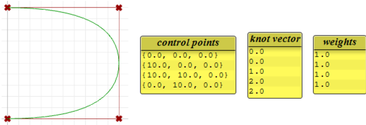
图44: 分析三阶开放非有理NURBS曲线
