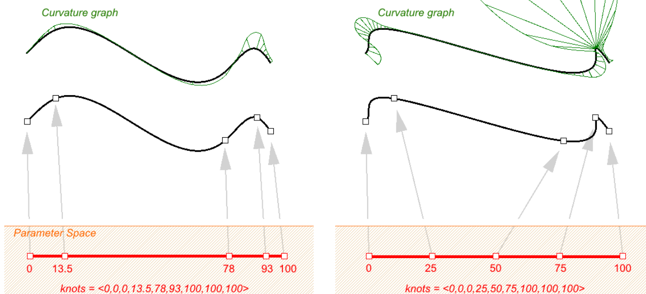
图41：非均匀节点列表可以帮助平滑曲线
